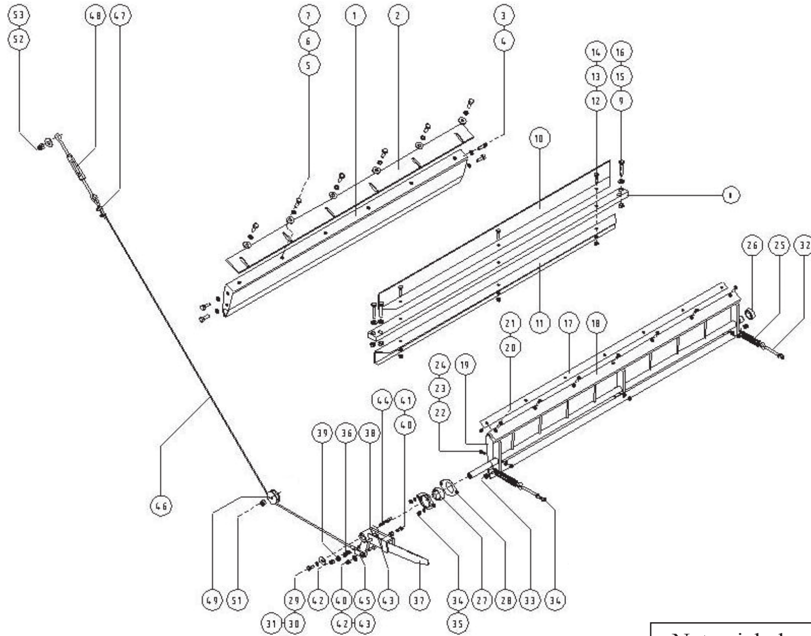
Netzwickelvorrichtung
