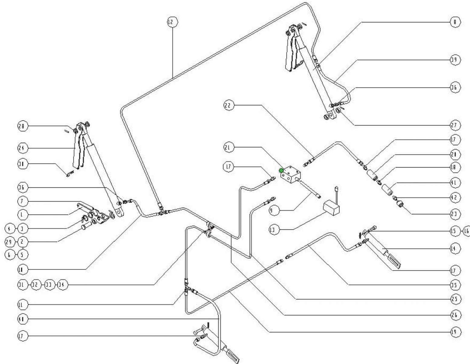
Hydraulikanlage
