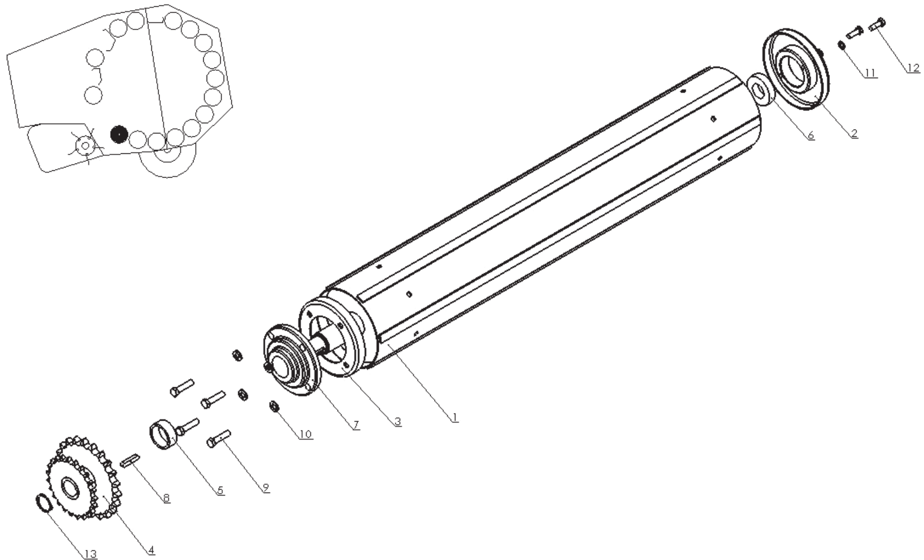
Rollwalze komplett VI
