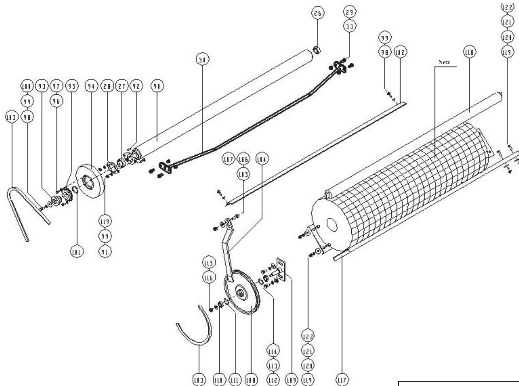
Netzwickelvorrichtung
