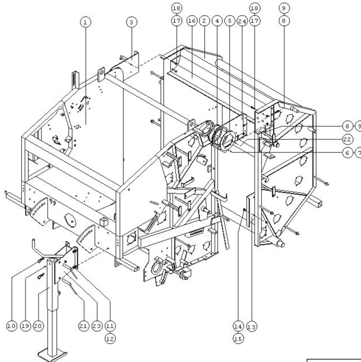
Pressengehäuse komplett
