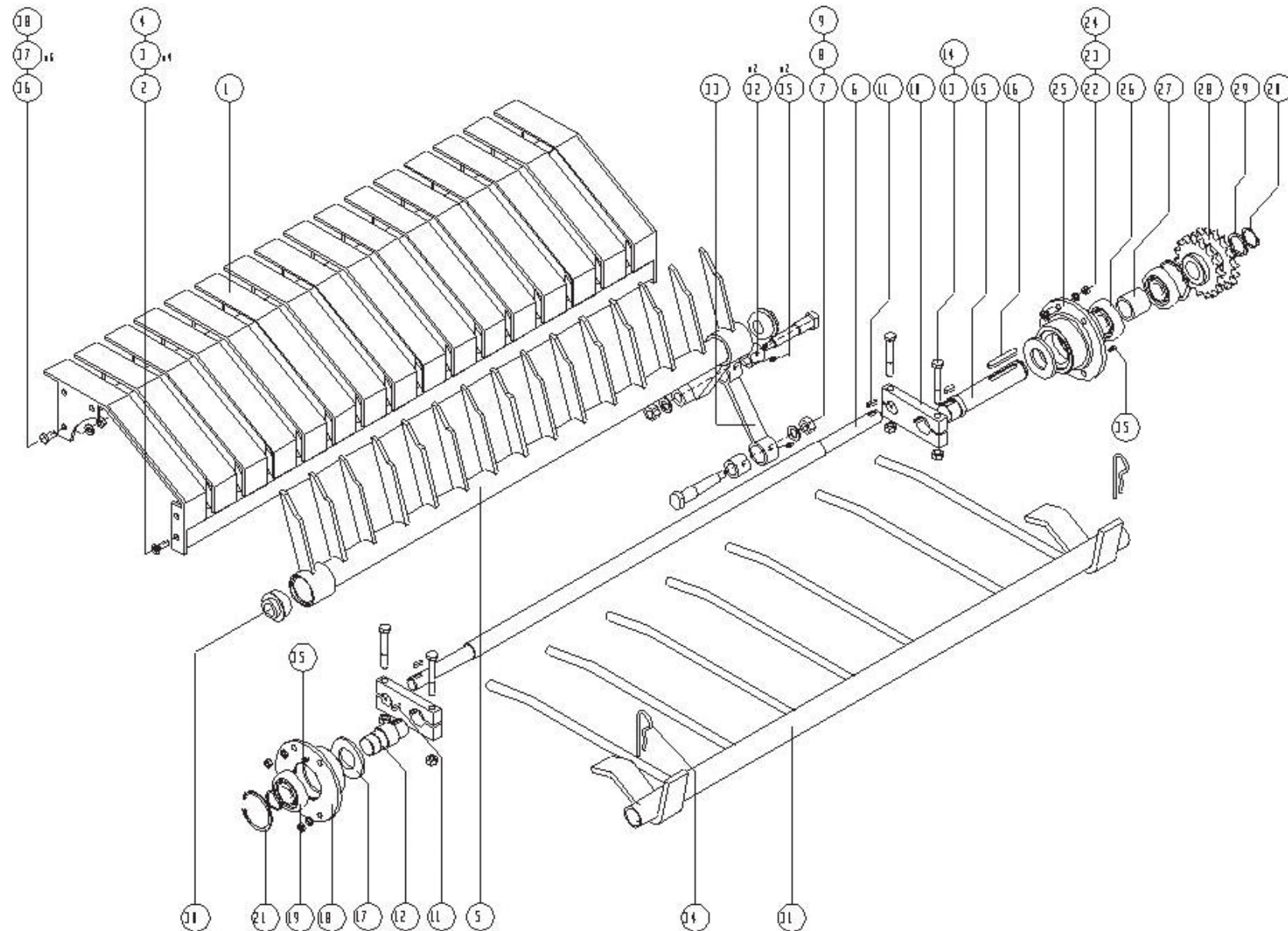
Wurfvorrichtung komplett
