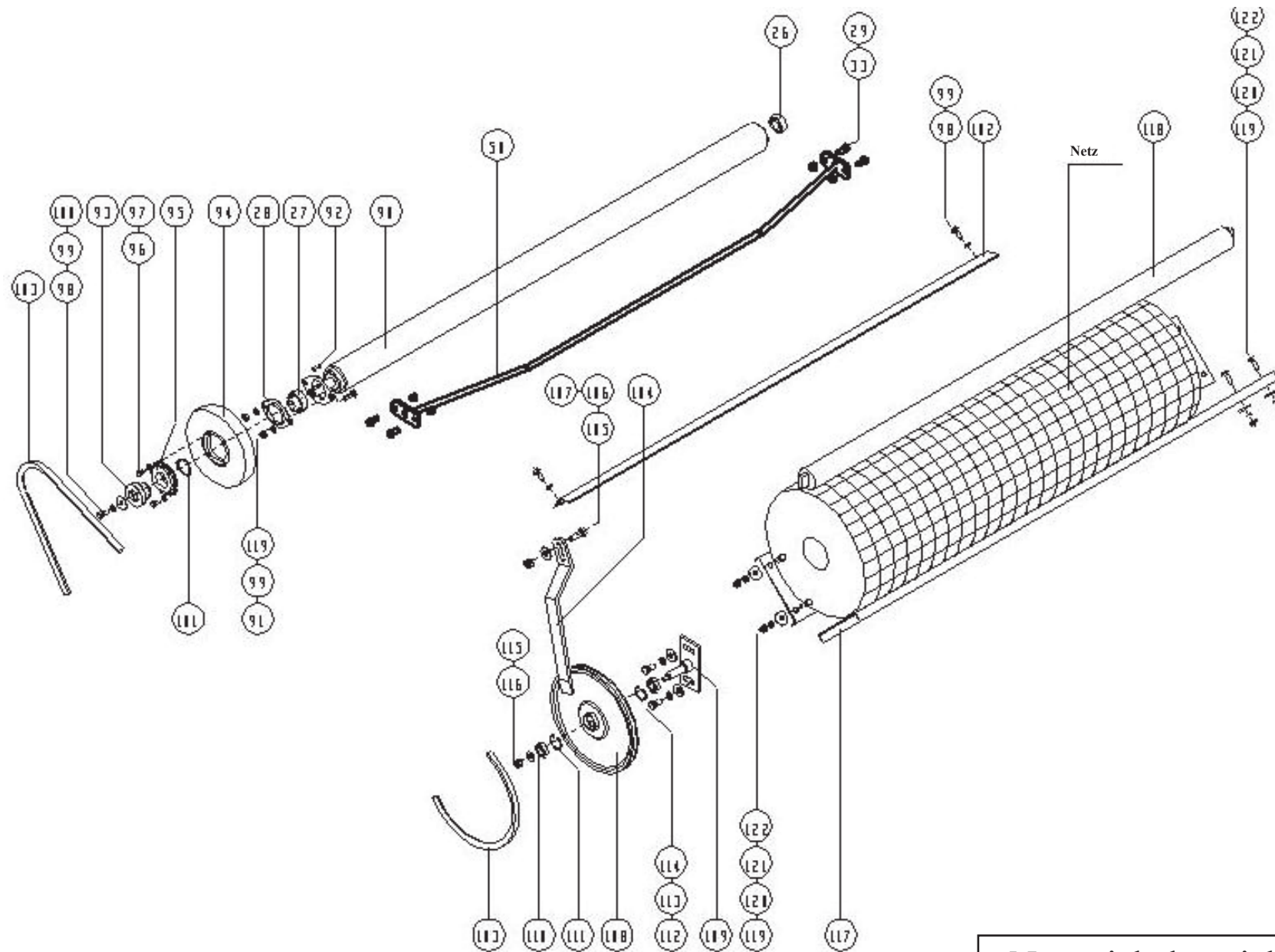
Netzwickelvorrichtung
