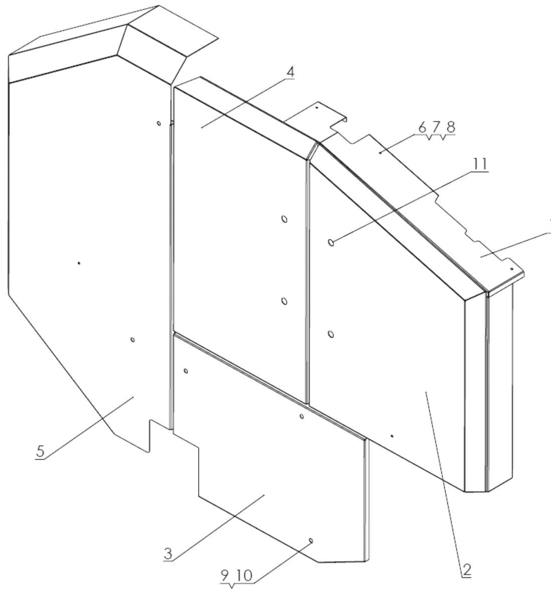
Abgesicherte rechte Abdeckungen
