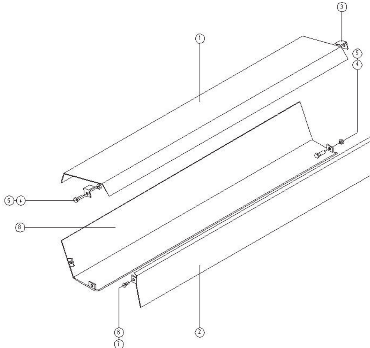
Abdeckungen der Seilwickelvorrichtung
