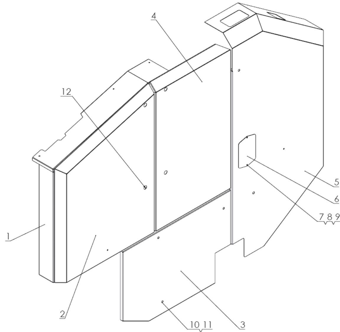
Abgeschernte linke Seitenabdeckungen
