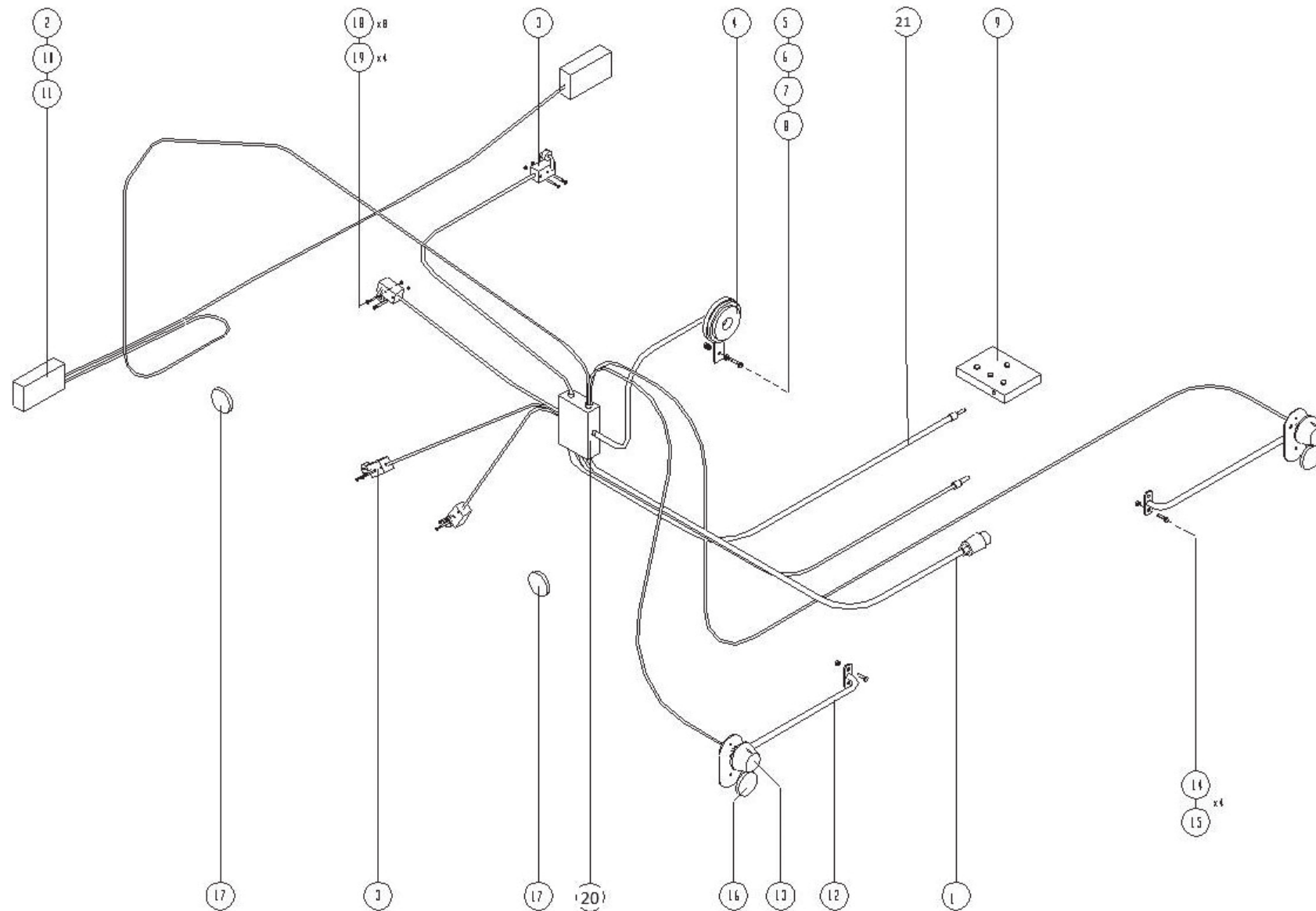
Elektroanlage
