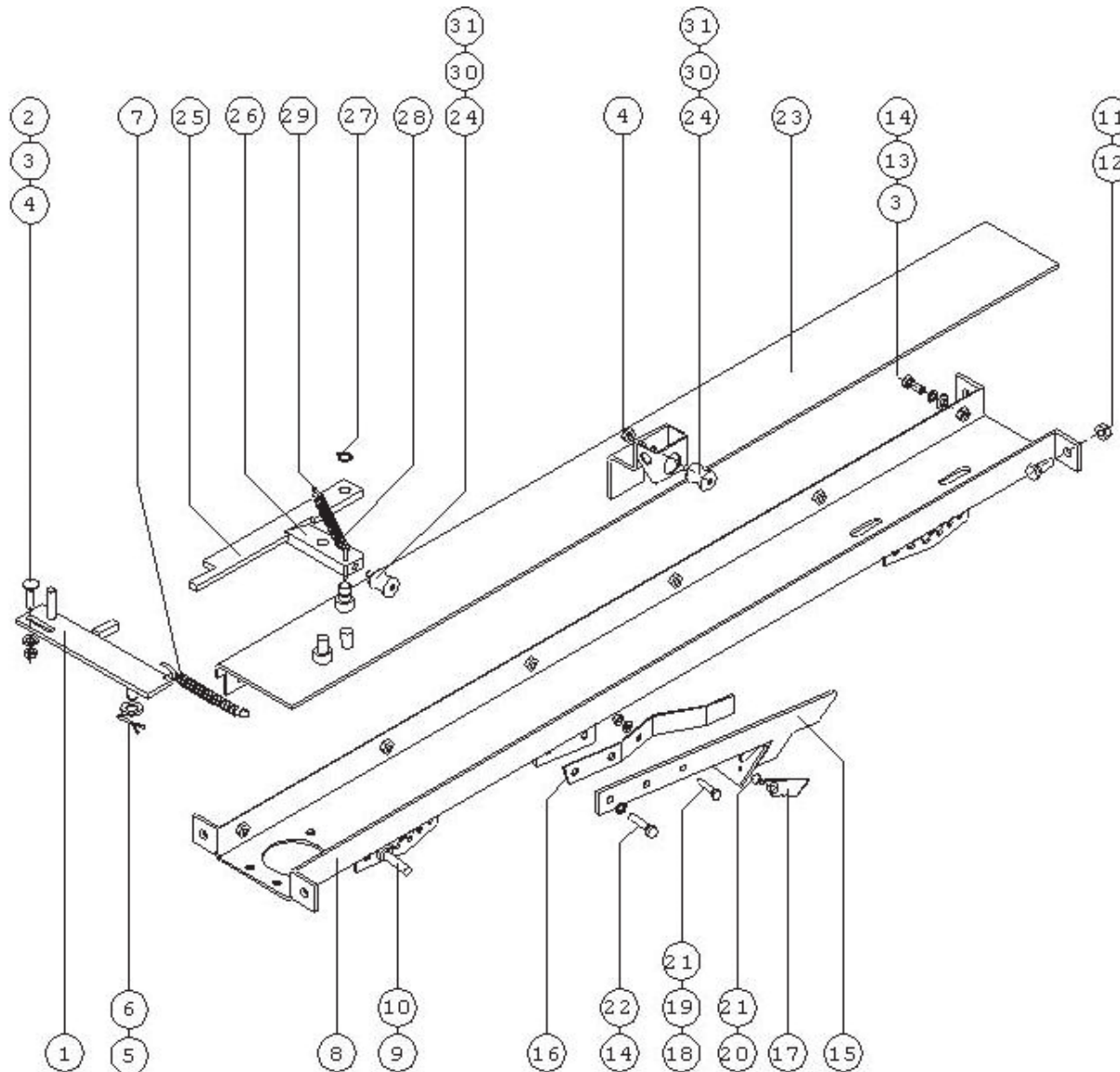
Gehäuse der Seilumwickelvorrichtung
