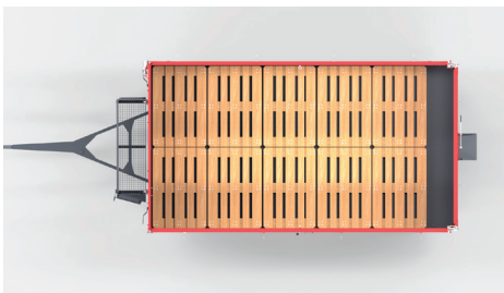
Długość przestrzeni ładunkowej wynosi 4190mm. Szerokość paletowa 2080mm Możliwość ustawienia 10 europalet
