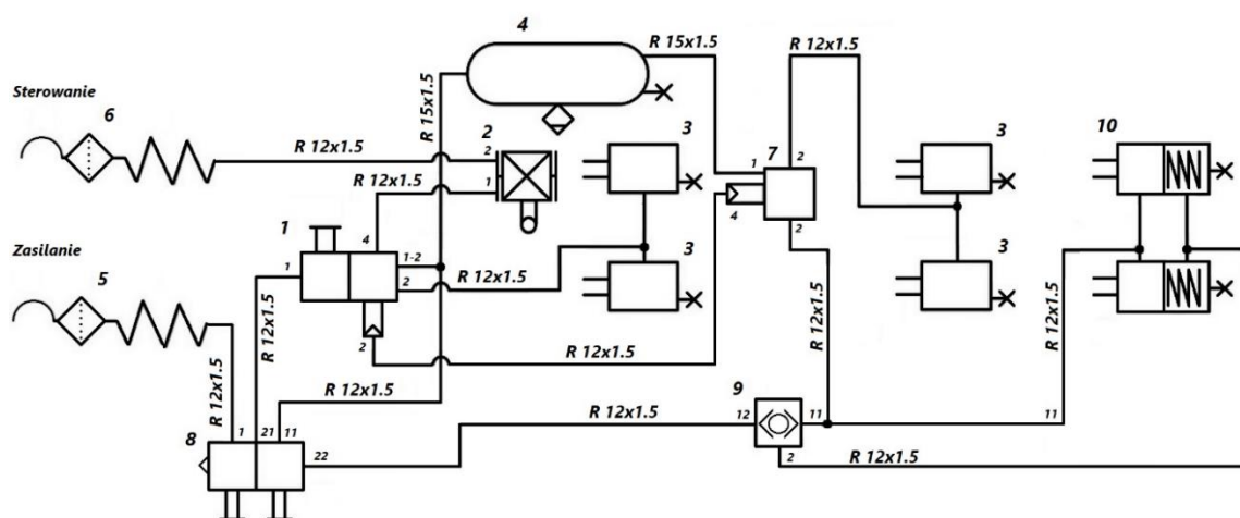
Rysunek 16. Instalacja hamulcowa pneumatyczna z ALB i zaworem parkująco - luzującym przyczepej dwu - osiowej.
