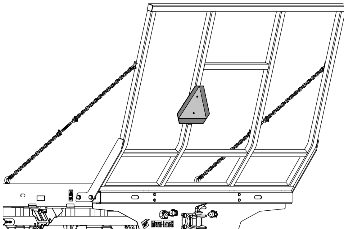
Rysunek 20. Umieszczenie trójkąta wyróżniającego pojazdy wolno poruszające się.
