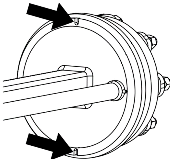
Rysunek 26. Miejsc kontroli zużycia okładzin hamulcowych.
