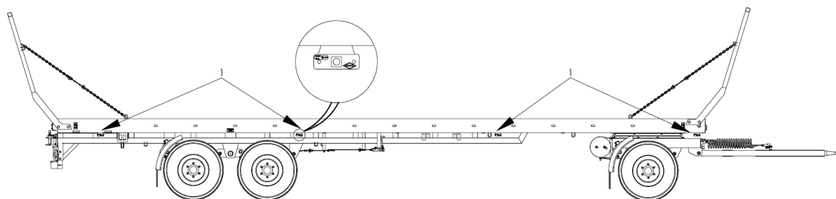
Rysunek 13. Rozmieszczenie elementów instalacji elektrycznej z prawej strony (strona lewa jest symetryczna): 1 – lampa obrysowa.
