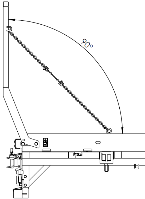
Rysunek 21. Ustawienie tylnej ściany oporowej podczas jazdy po drogach publicznych.
