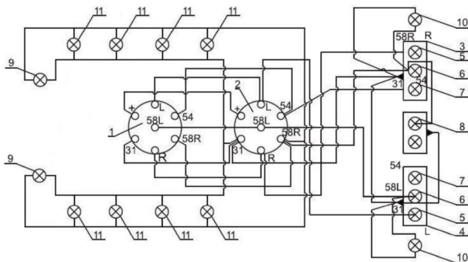
Rysunek 10. Schemat instalacji oświetleniowej: 1 - wtyczka 7 kontaktowa, 2 - gniazdo 7 kontaktowe, 3 - tylna lampa zespolona prawa, 4 - tylna lampa zespolona lewa, 5 - żarówki świateł, kierunku jazdy, 6 - żarówki świateł pozycyjnych tylnych, 7 - żarówki świateł hamowania "STOP", 8- żarówki światła oświetlenia tablicy rejestracyjnej, 9 - lampa światła pozycyjnego przedniego, 10 - lampa światła obrysowego, 11- lampa światła obrysowego bocznego.
