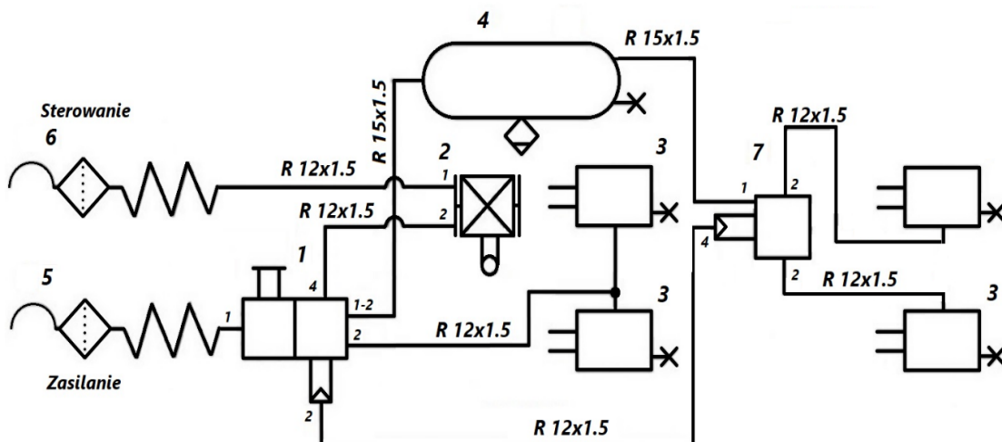
Rysunek 14. Instalacja hamulcowa pneumatyczna z ALB przyczepy dwu - osiowej.
