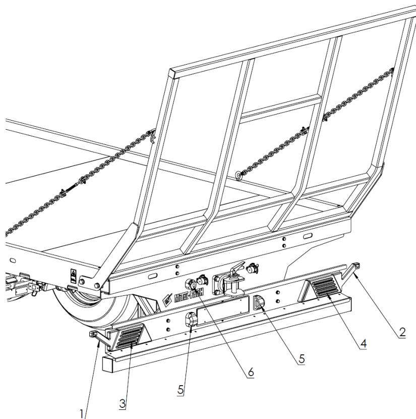
Rysunek 12. Rozmieszczenie elementów instalacji elektrycznej: (1) – lampa obrysowa lewa, (2) – lampa obrysowa prawa, (3) – lampa zespolona lewa, (4) – lampa zespolona prawa, (5) – oświetlenie tablicy rejestracyjnej, (6) – gniazdo przyłączeniowe.
