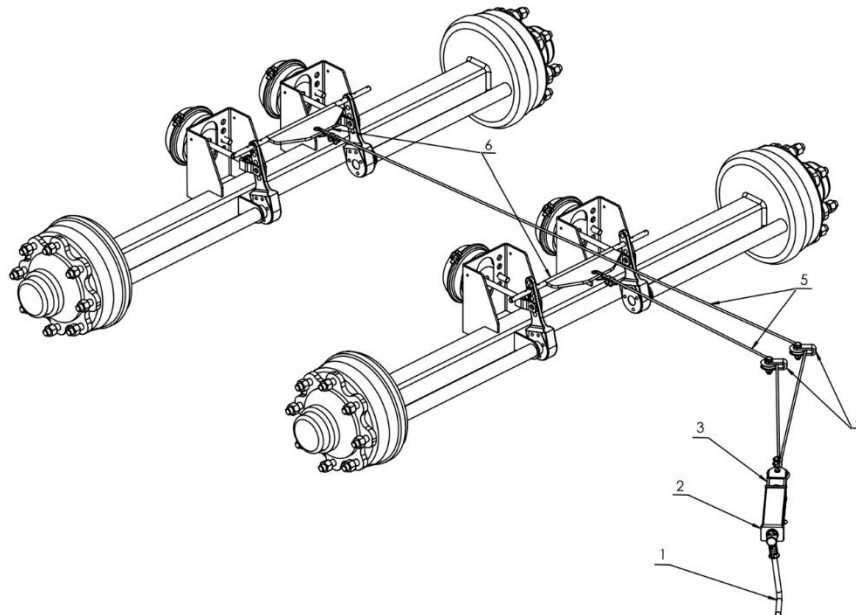
Rysunek 18. Instalacja hamulca postojowego ręcznego: 1 – korbka, 2 – obudowa, 3 – naciąg, 4 – rolki prowadzące, 5 – linka stalowa, 6 – poprzeczka hamulca.
