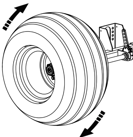
Rysunek 22. Sprawdzenie luzu łożysk kół.
