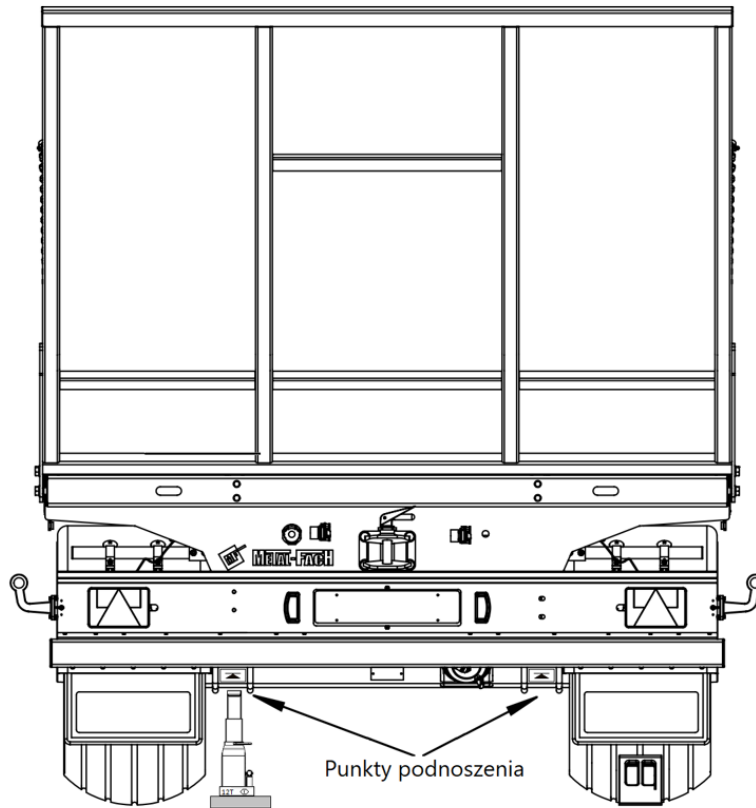
Rysunek 23. Punkty podparcia podnośników. Strzałki wskazują miejsca w których dozwolone jest umieszczenie podnośnika.
