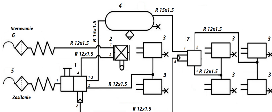
Rysunek 15. Instalacja hamulcowa pneumatyczna z ALB przyczepej trzy - osiowej.
