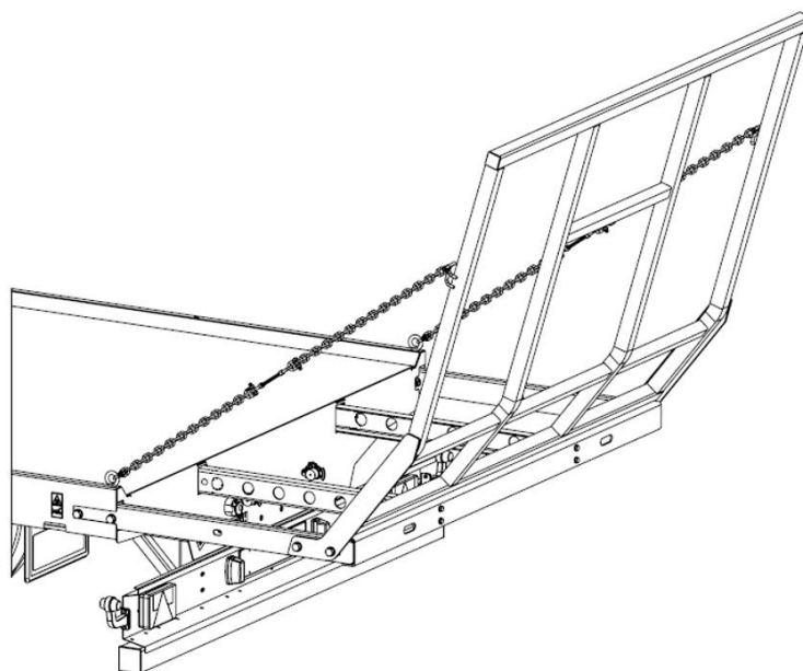
Rysunek 9. Rama wydłużająca przestrzeń ładunkową
