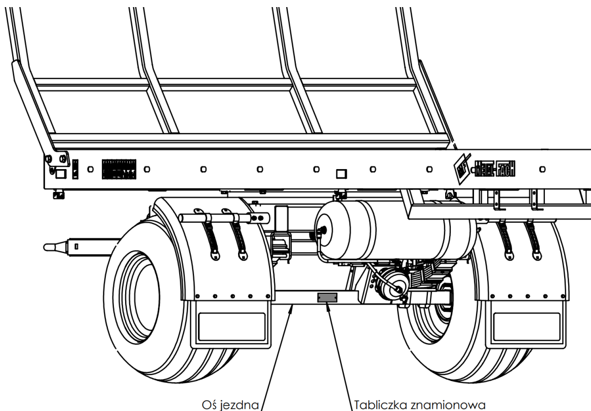
Rysunek 3. Umiejscowienie tabliczki znamionowej na osi jezdnej.
