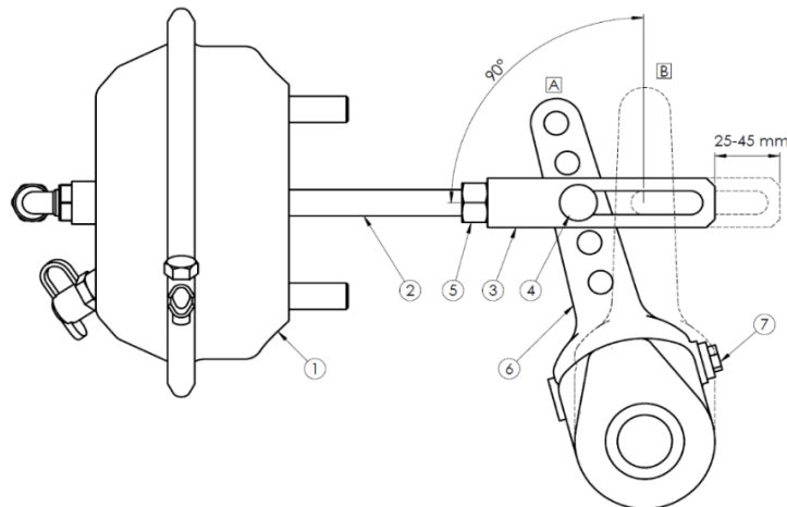
Rysunek 27. Regulacja hamulca zasadniczego. 1 – siłownik pneumatyczny, 2 – tłoczysko siłownika, 3 – widełki siłownika, 4 – sworzeń widełek, 5 – nakrętka blokująca widełka, 6 – dźwignia rozpieraka, 7 – śruba regulacyjna: A – położenie dźwigni w pozycji odhamowanej, B – położeni dźwigni w pozycji zahamowanej.
