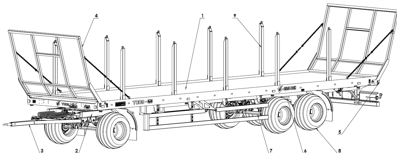
Rysunek 8. Budowa przyczep: rama (1), wózek obrotnicy (2), dyszel (3), ściana oporowa (4), rama wysuwana (5), zawieszenie (6), oś jezdna (7), koło (8), opcjonalne kłonicie (9)
