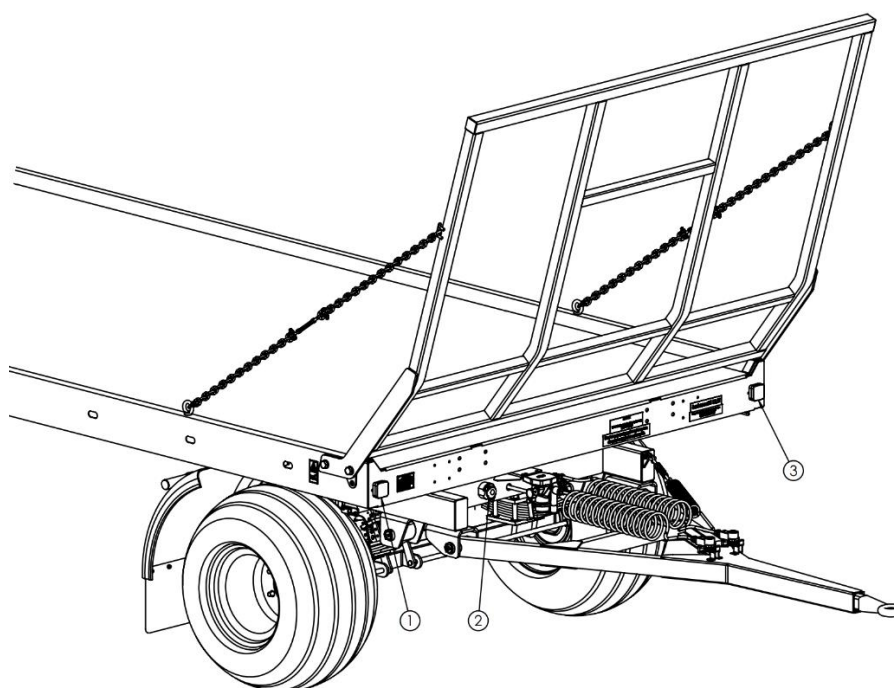
Rysunek 11. Rozmieszczenie elementów instalacji elektrycznej z przodu: 1 - lampa obrysowa prawa, 2 - gniazdo przyłączeniowe, 3 - lampa obrysowa lewa.
