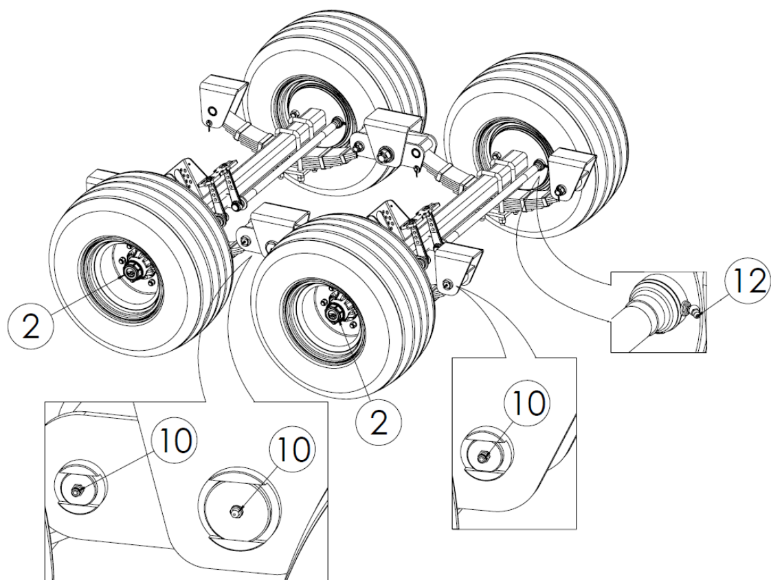
Rysunek 52. Punkty smarne zawieszenia tandem dla wozu paszowego BEL-MIX T659/4
