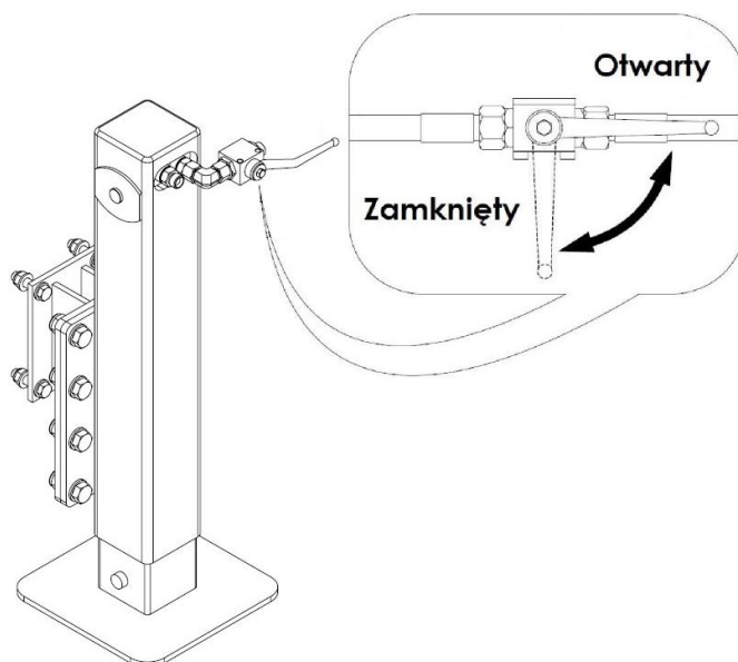
Rysunek 36. Zawór hydrauliczny sterujący (odcinający) stopkę hydrauliczną
