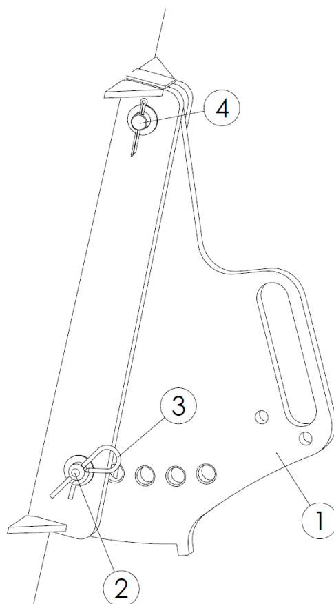
Rysunek 40. Przeciwnóż ręczny: 1 – przeciwnóż, 2 – sworzeń dolny, 3 – zawleczka, 4 – sworzeń górny
