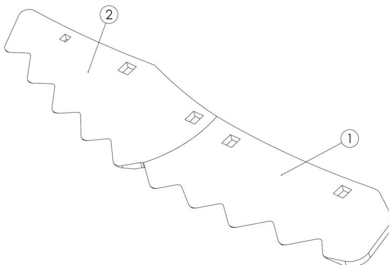
Rysunek 61. Ostrzenie noży: 1 – nóż tnący I, 2 - nóż tnący II
