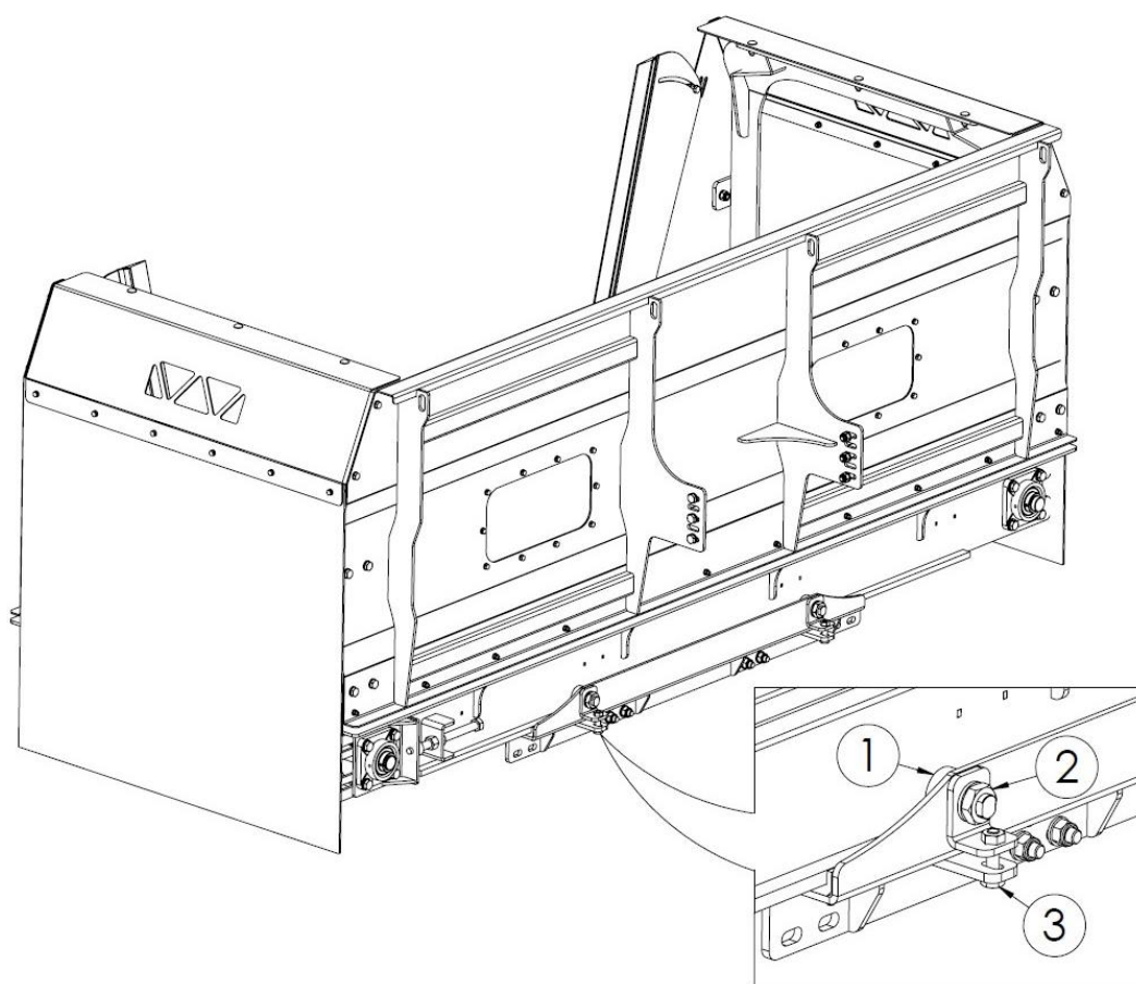
Rysunek 58. Naciąg łożysk przesuwu: 1- łożysko, 2 – nakrętka, 3 - śruba naciągu
