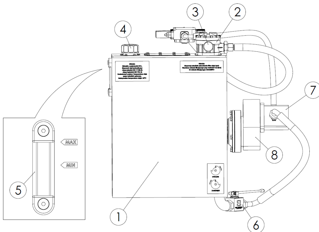
Rysunek 48. Hydraulika własna: 1 – zbiornik oleju, 2 – filtr, 3 – wskaźnik zabrudzenia, 4 – wlew oleju, 5 – wskaźnik poziomu oleju, 6 – zawór kulowy, 7 – pompa hydrauliczna, 8 – multiplikator
