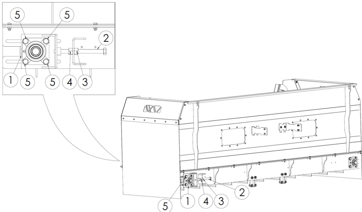
Rysunek 56. Napinanie taśmy podajnika: 1 – naciąg, 2 – śruba naciągu, 3 – nakrętka naciągu, 4 – nakrętka, 5- połączenie śrubowe łożyska wałka podajnika
