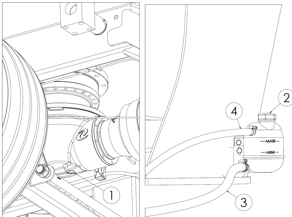
Rysunek 54. Wymiana oleju przekładni planetarna: 1 – korek spustowy, 2 – korek zbiorniczka wyrównawczego, 3 – przewód zasilający, 4 – przewód odpowietrzający
