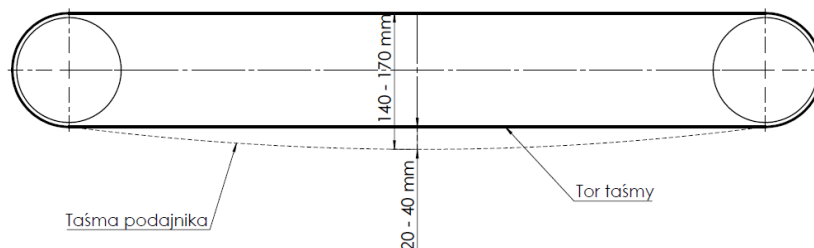
Rysunek 57. Sprawdzenie naciągu taśmy
