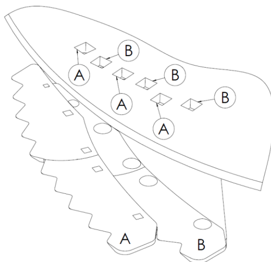
Rysunek 60. Zmiana położenia noży tnących: A – noże tnące wysunięte, B – noże tnące schowane
