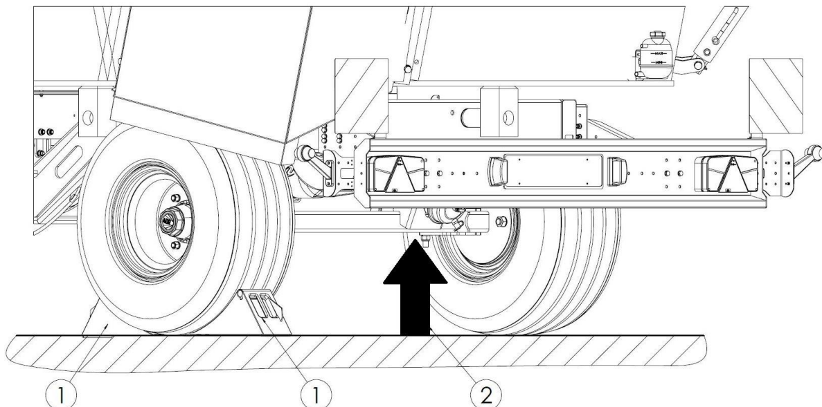
Rysunek 44. Punkty przyłożenia podnośnika: 1 – kliny, 2 – podnośnik
