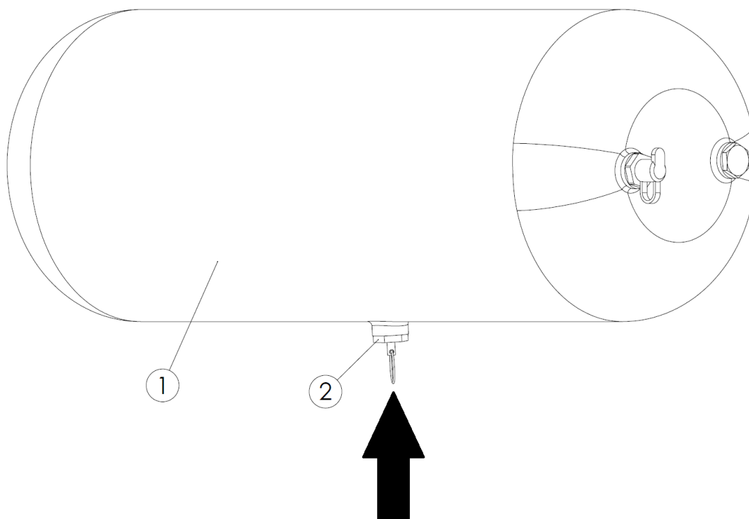
Rysunek 47. Odwadnianie zbiornika powietrza: 1 - zbiornik powietrza, 2 - zawór odwadniający
