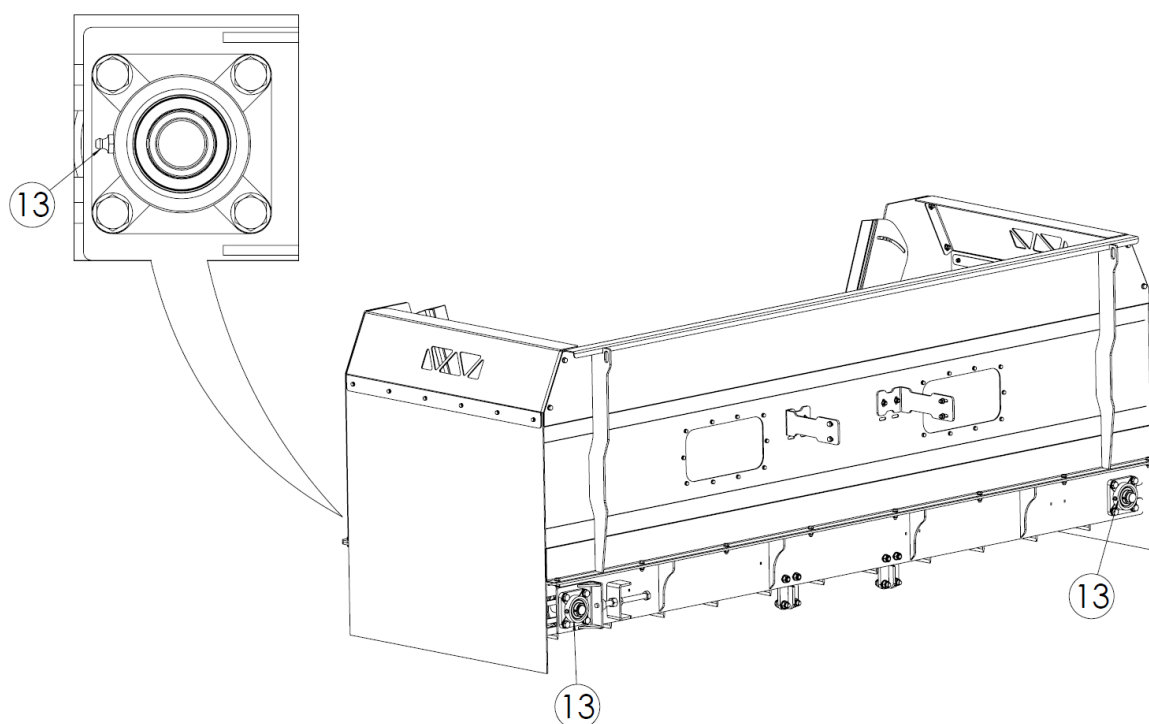
Rysunek 53. Punkty smarne podajnik
