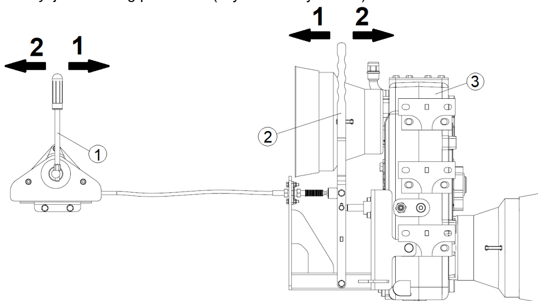
Rysunek 39. Zmiana przełożenia w przekładni dwubiegowej: 1 – dźwignia zmiany przełożenia, 2 – dźwignia zmiany przełożenia przy przekładni, 3 – przekładnia dwubiegowa
