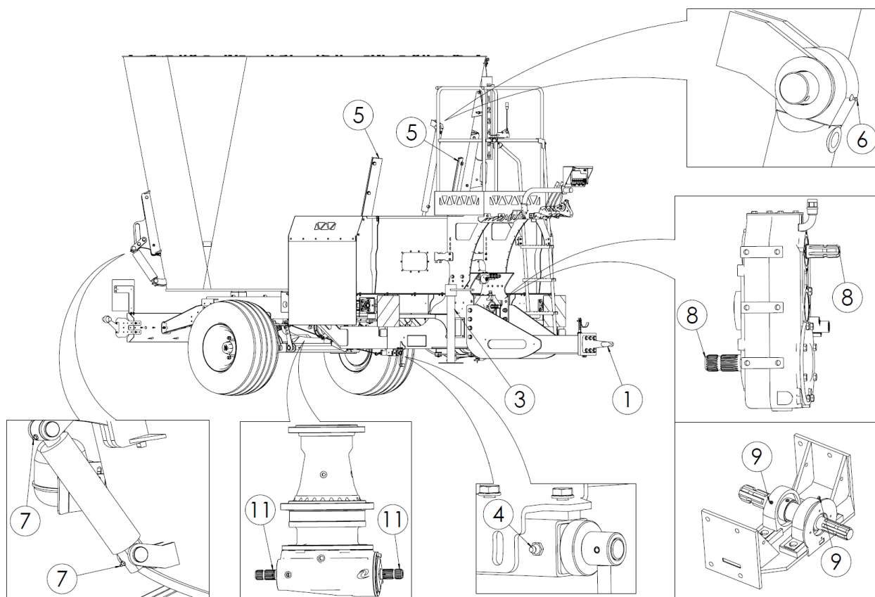
Rysunek 50. Punkty smarne wozu paszowego
