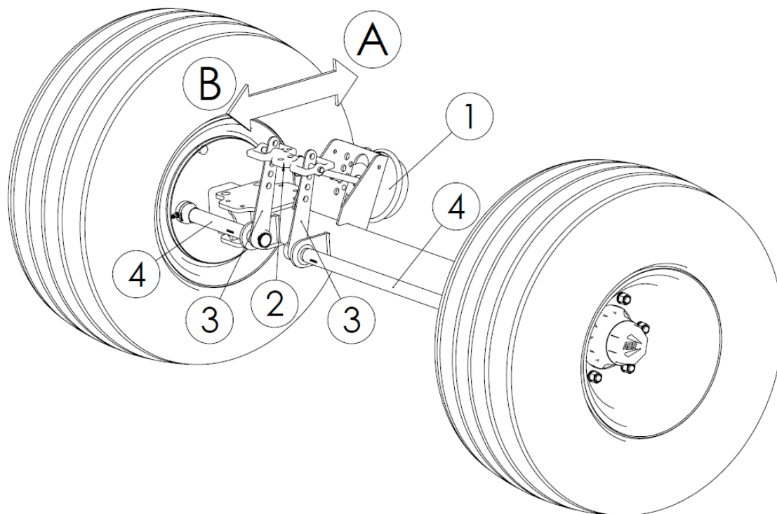
Rysunek 43. Regulacja hamulca zasadniczego
