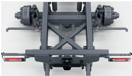
Zastrzały krzyżowe w tylnej części ramy - wzmocnienie osi wywrotu
