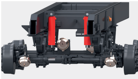
Stabilizacja hydrauliczna osi
