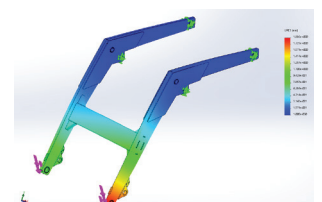
Obliczenia wytrzymałościowe - MES
