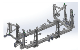
Projektowanie przyrządów dedykowanych (spawanie, obróbka skrawaniem, gięcie)
