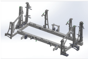
Projektowanie przyrządów w systemie CAD
