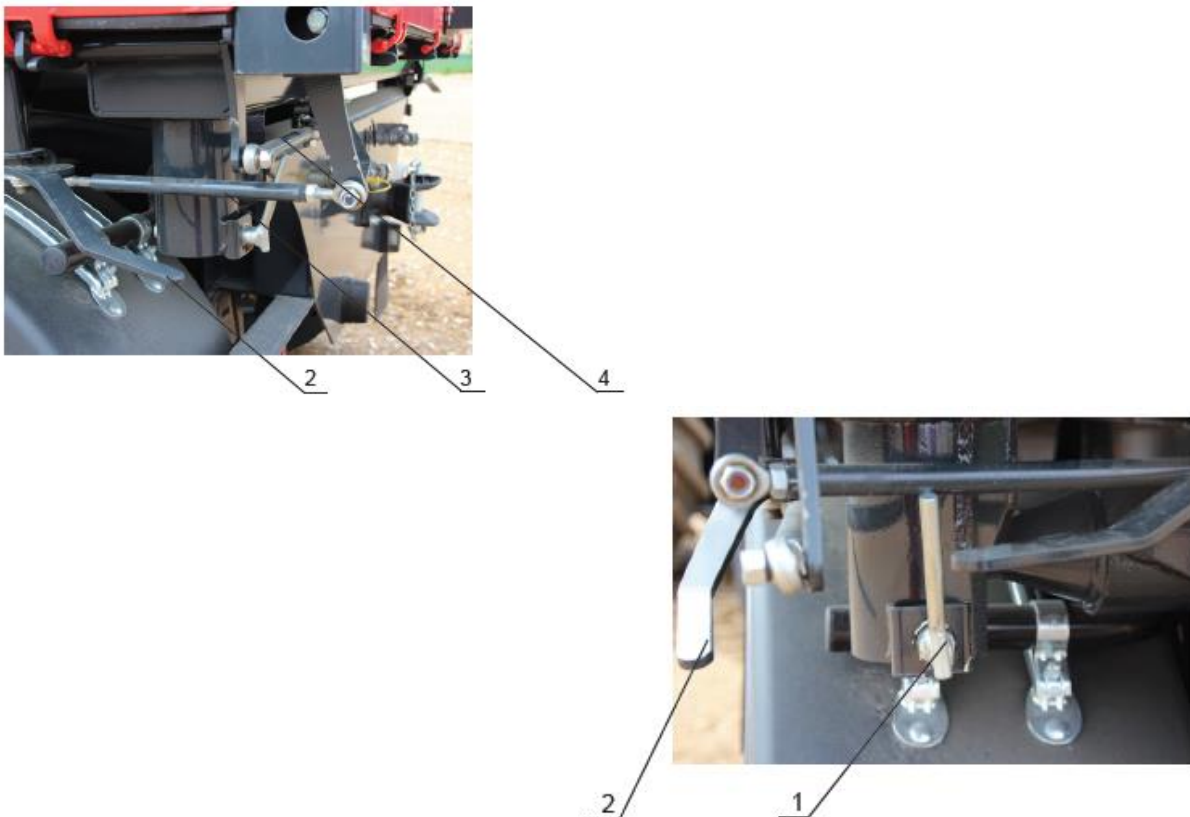
Rysunek 14. Zamki ścian skrzyni ładunkowej.
