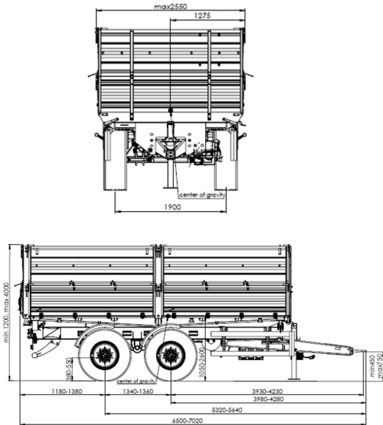
Rysunek 9. Wymiary gabarytowe przyczepy T959
