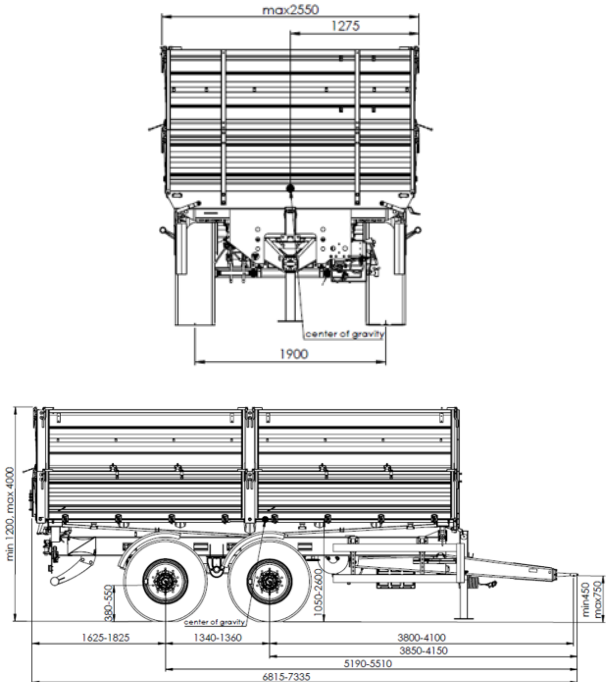
Rysunek 8. Wymiary przyczepy gabarytowe przyczepy T755A
