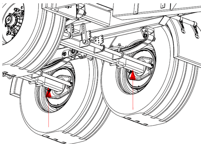
Rysunek 7. Miejsce przyłożenia podnośników
