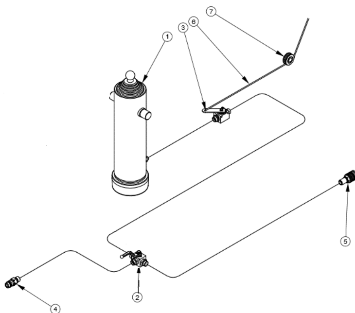
Rysunek 10. Schemat instalacji hydraulicznej mechanizmu przechylenia skrzyni ładunkowej: 1 - siłownik, 2 – zawór przełączający, 3 - zawór odcinający, 4 – wtyczka zaworu złącznego, 5 - gniazdo zaworu złącznego, 6 – linka sterująca zaworem odcinającym, 7- rolka linki
