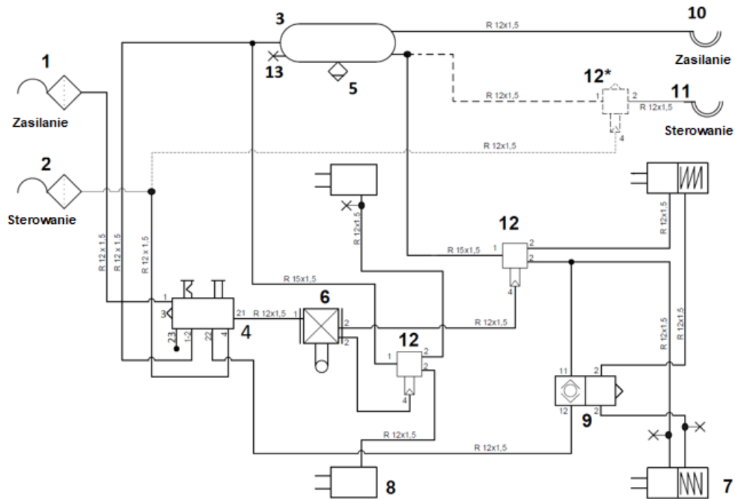
Rysunek 13. Schemat pneumatycznej instalacji hamulcowej dwuprzewodowej – siłowniki membranowo – sprężynowe:
