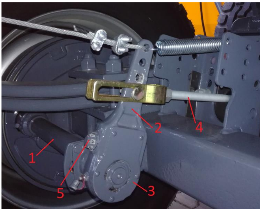
Rysunek 15. Elementy układu hamulcowego:
