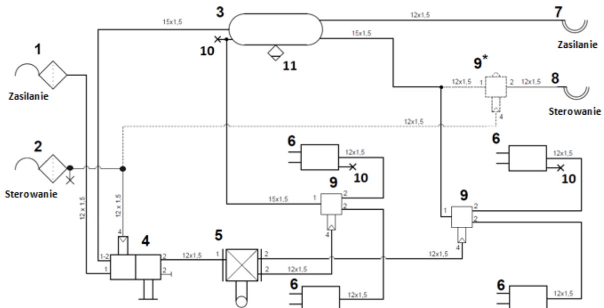
Rysunek 12. Schemat pneumatycznej instalacji hamulcowej dwuprzewodowej – siłowniki membranowe:
