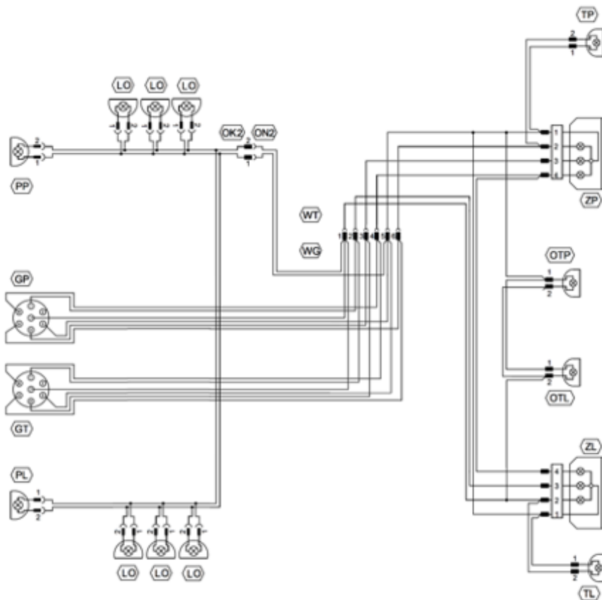
Rysunek 11. Schemat instalacji elektrycznej przyczepy:
