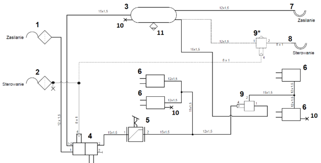
Rysunek 15. Schemat dwuprzewodowej pneumatycznej instalacji hamulcowej – regulator ręczny:
