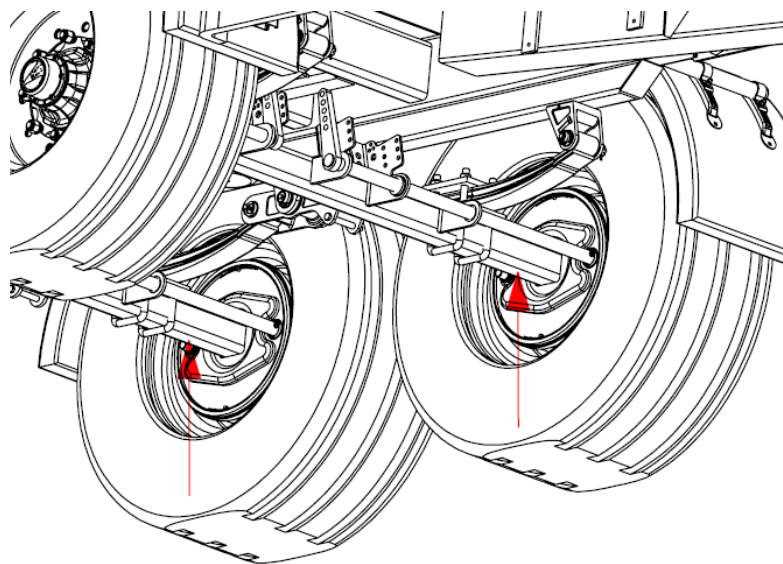
Rysunek 8. Miejsce przyłożenia podnośników
