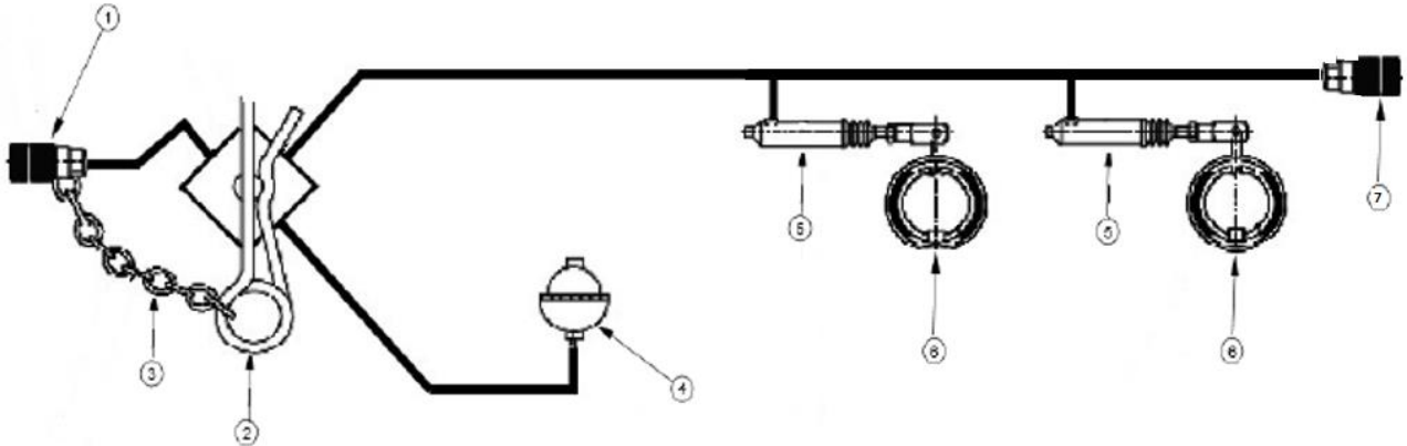
Rysunek 16. Schemat hydraulicznej instalacji hamulcowej:
