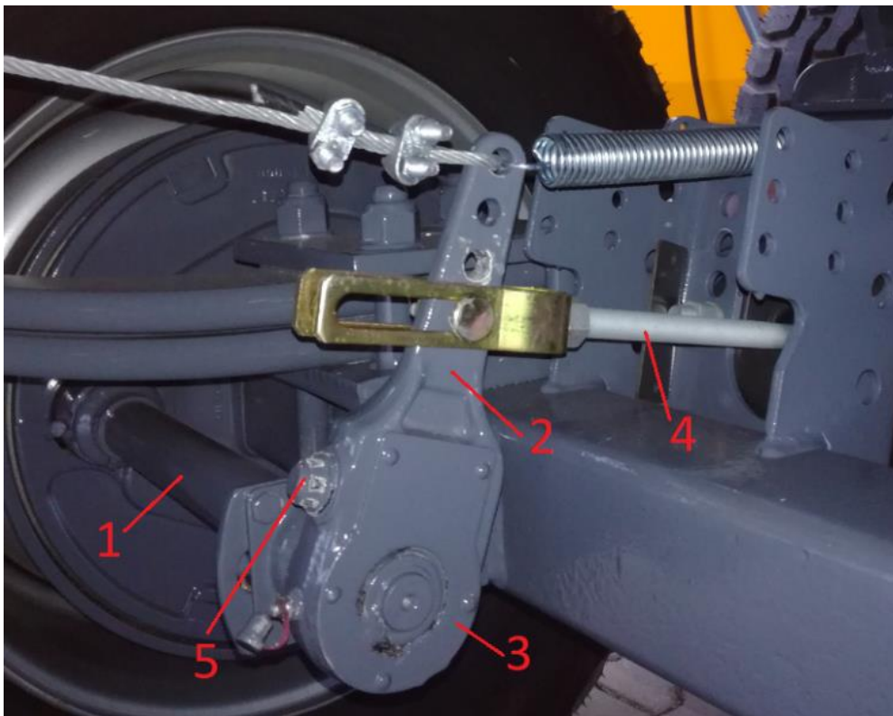
Rysunek 18. Elementy układu hamulcowego: 1-walek rozpieraka szczęk, 2-dźwignia (ramię) wałka rozpieraka, 3-zębátka na wałku rozpieraka, 4-ciężno (popychacz) łączące tłocznisko siłownika pneumatycznego z ramieniem wałka rozpieraka, 5 - śruba regulacji
