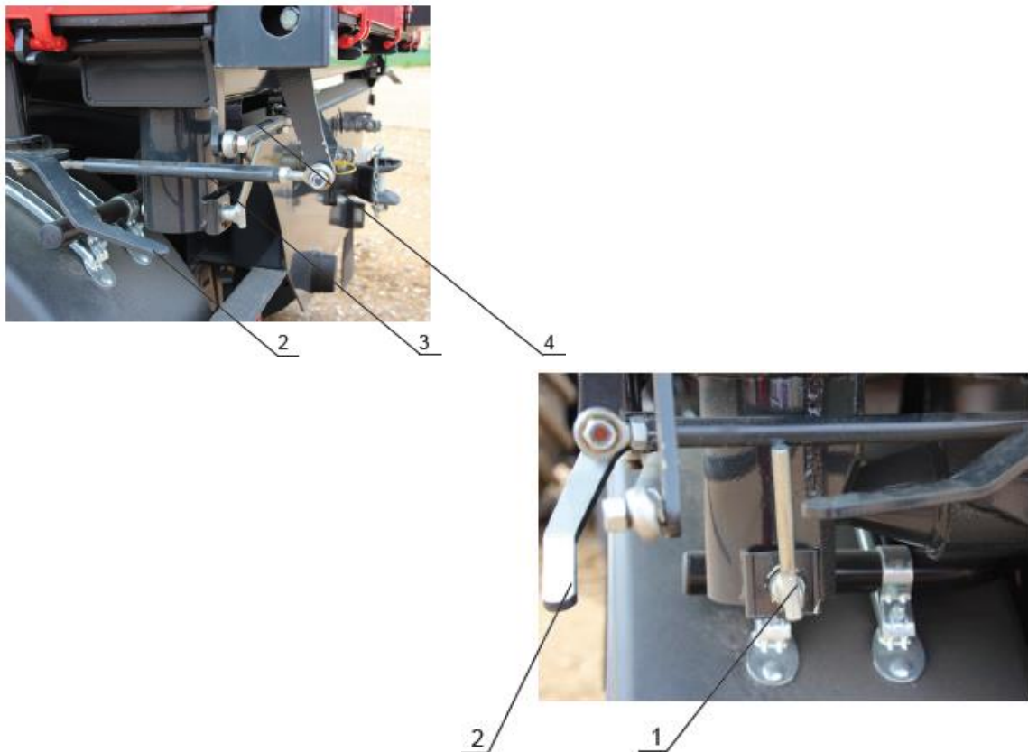
Rysunek 17. Zamki ścian skrzyni ładunkowej: 1- sworznie wywrotu, 2 - dźwignia centralna zamków dolnych, 3 – ciągnio boczne zamków, 4 – ciągnio tylne zamków
