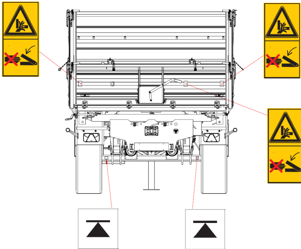
Rysunek 5. Rozmieszczenie piktogramów na ścianach przyczepy – tył
