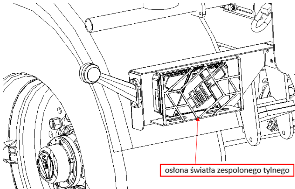
Rysunek 13. Umiejscowienie osłony światła zespolonego tylnego
