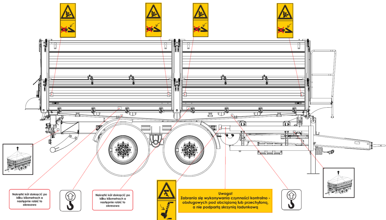
Rysunek 6. Rozmieszczenie piktogramów na ścianach przyczepy – strona prawa
