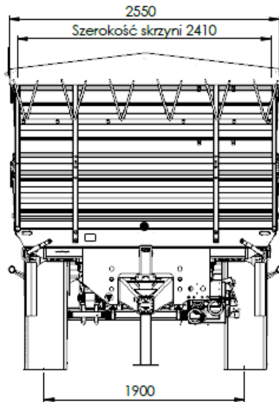
Rysunek 9. Wymiary przyczepy – widok z przodu
