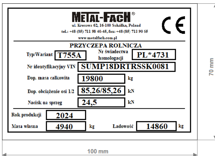
Rysunek 2. Przykładowa tabliczka znamionowa
