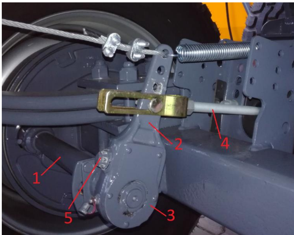
Rysunek 20. Elementy układu hamulcowego: 1-walek rozpieraka szczęk, 2-dźwignia (ramię) wałka rozpieraka, 3-zębátka na wałku rozpieraka, 4-ciężno (popychacz) łączące tłocznisko siłownika pneumatycznego z ramieniem wałka rozpieraka, 5 - śruba regulacji
