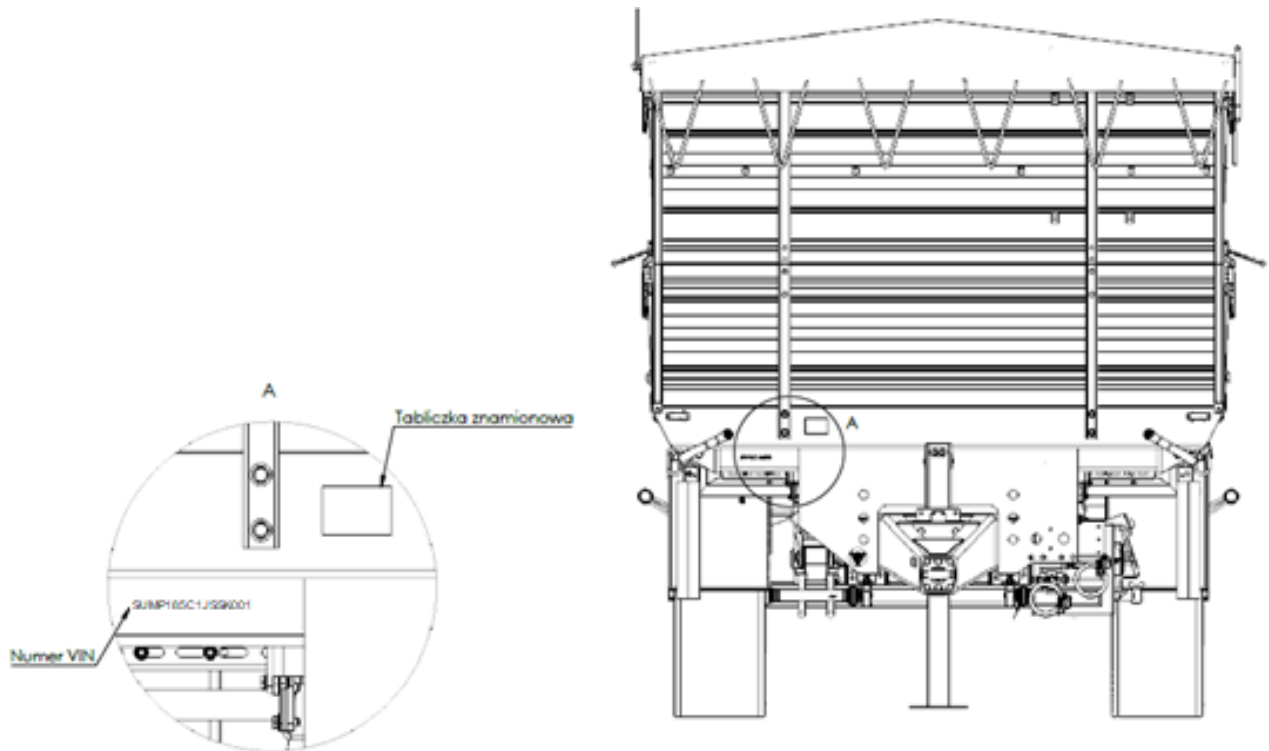
Rysunek 1. Umieszczenie tabliczki znamionowej oraz numeru VIN na maszynie
