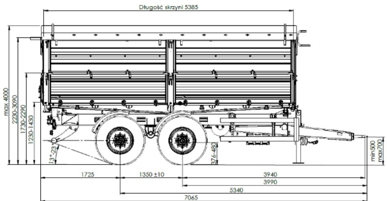
Rysunek 10. Wymiary przyczepy – widok z boku
