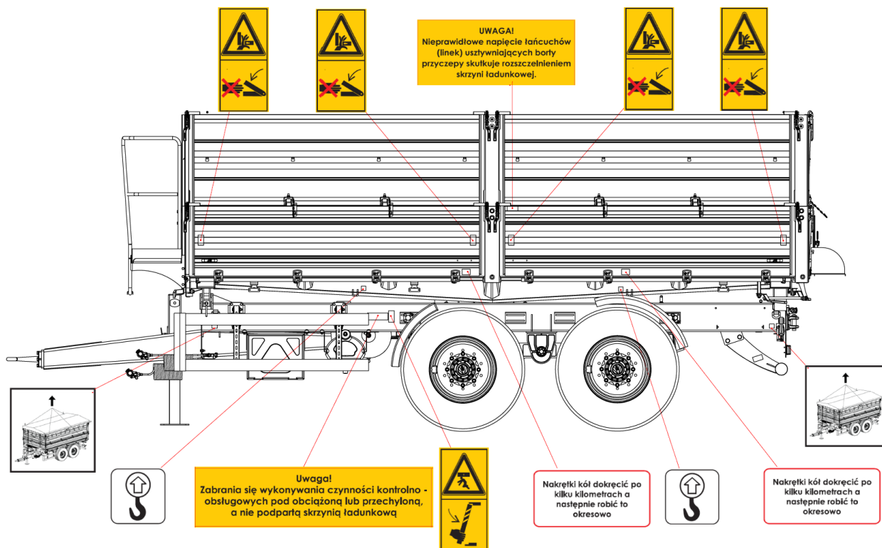
Rysunek 7. Rozmieszczenie piktogramów na ścianach przyczepy – strona lewa
