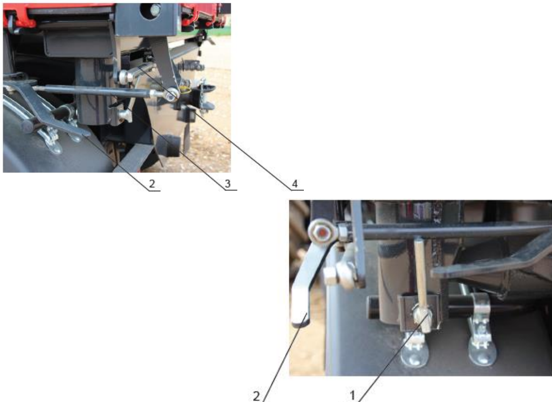
Rysunek 19. Zamki ścian skrzyni ładunkowej: 1- sworznie wywrotu, 2 - dźwignia centralna zamków dolnych, 3 – ciągnio boczne zamków, 4 – ciągnio tylne zamków
