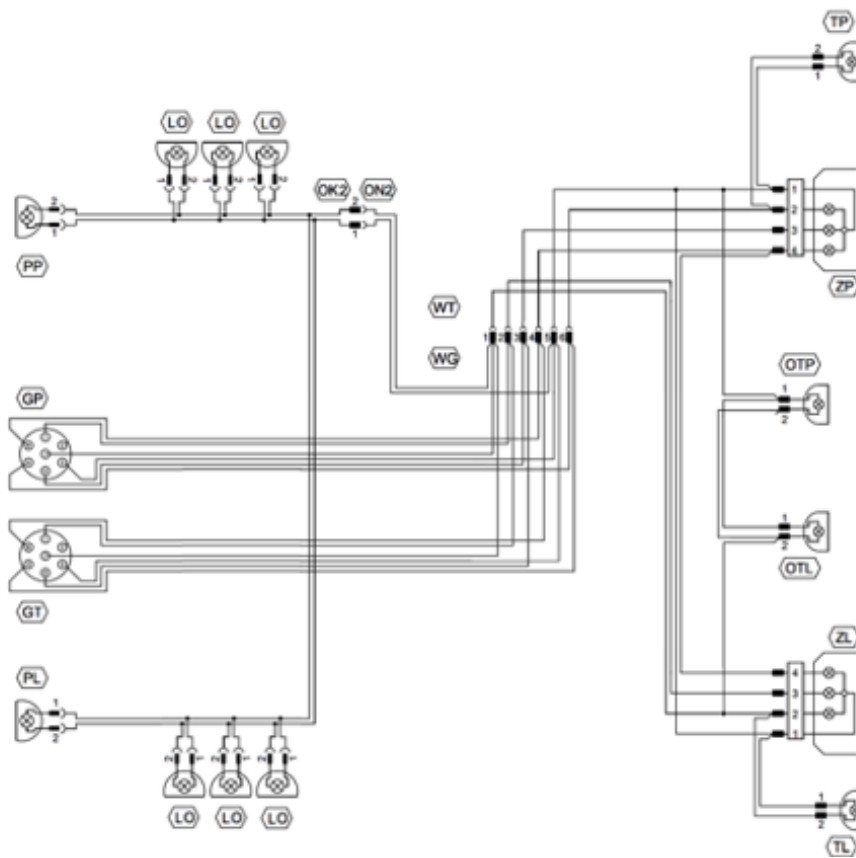
Rysunek 12. Schemat instalacji oświetleniowej:
