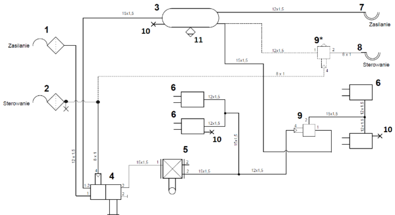
Rysunek 14. Schemat dwuprzewodowej pneumatycznej instalacji hamulcowej – regulator automatyczny (ALB):
