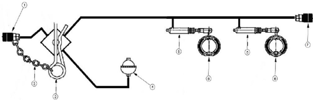
Rysunek 16. Schemat hydraulicznej instalacji hamulcowej:
