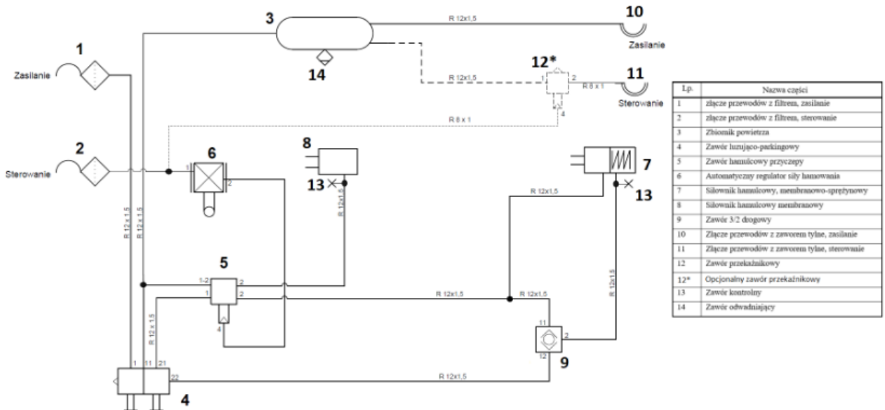
Rysunek 19. Schemat instalacji z siłownikami membranowo-sprężynowymi bez zaworu przełącznikowego – hamulec postojowy
