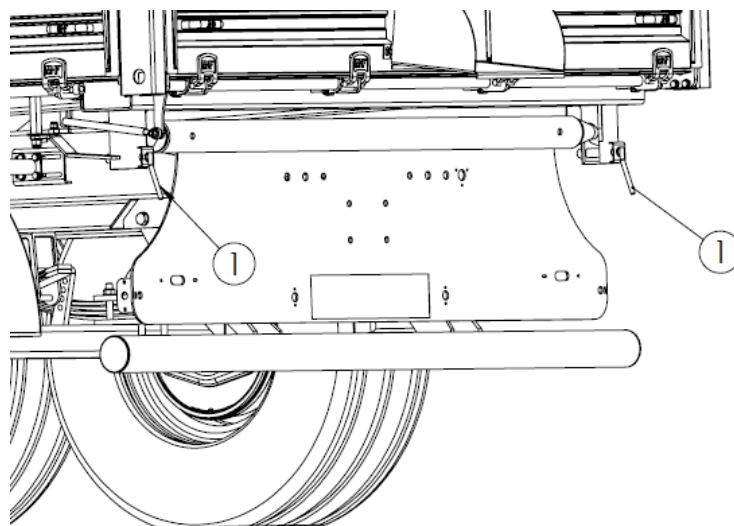
Rysunek 23. Sworznie zabezpieczające wywrotu
