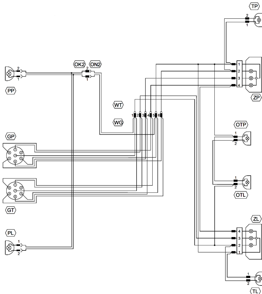
Rysunek 11. Schemat instalacji elektrycznej przyczepy bez światel pozycyjnych bocznych (wersja podstawowa): ZP - lampa zespolona tylna prawa, ZL - lampa zespolona tylna lewa, GP - gniazdo siedmiostykowe przednie, GT - gniazdo siedmiostykowe tylne, OTP - lampa oświetlenia tablicy rejestracyjnej prawa, OTL - lampa oświetlenia tablicy rejestracyjnej lewa, PP - lampa pozycyjna przednia prawa, PL - lampa pozycyjna przednia lewa, TP - lampa pozycyjna tylna prawa, TL - lampa pozycyjna tylna lewa. Oznaczenie połączeń gniazd GT oraz GP: 31 - masa + Zasilanie, L - kierunkowskaz lewy, 54 - światło STOP, 58L - tylne światło pozycyjne lewe, 58R - tylne światło pozycyjne prawe, R - kierunkowskaz prawy
