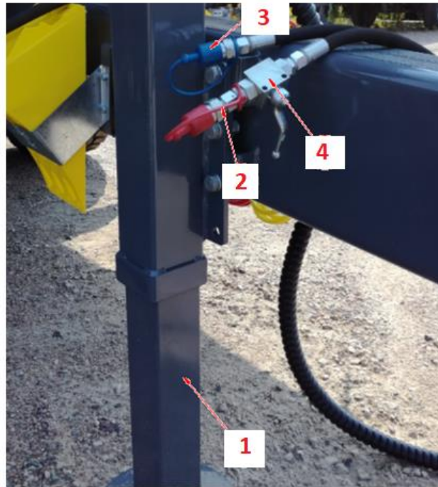
Rysunek 22. Stopka hydrauliczna. 1- stopka, 2- przewód zasilający, 3- przewód powrotu oleju, 4 – zawór odcinający
