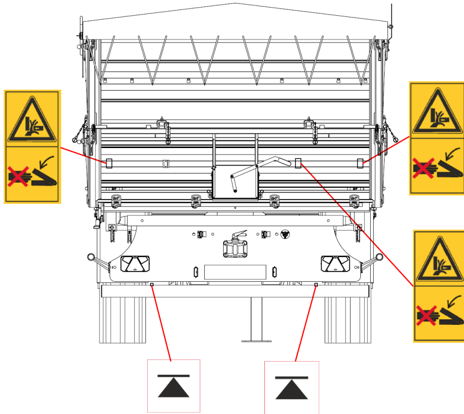
Rysunek 6. Rozmieszczenie piktogramów na ścianach przyczepy- tył
