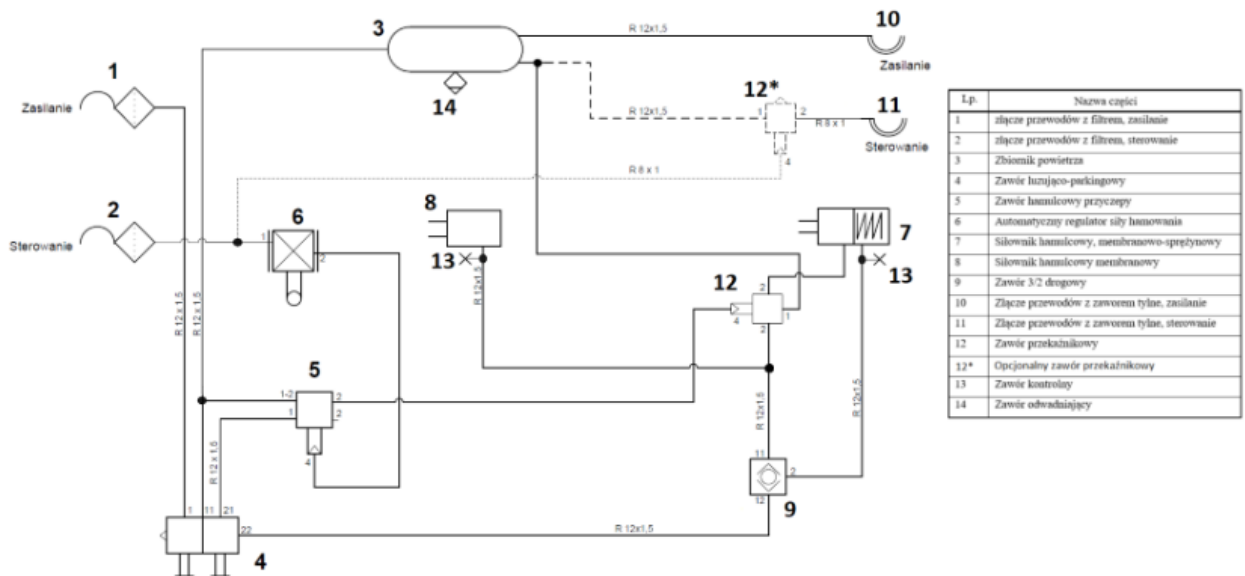
Rysunek 18. Schemat instalacji z siłownikami membranowo-sprężynowymi i zaworem przełącznikowym – hamulec postojowy
