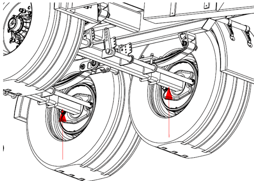
Rysunek 24. Miejsce przyłożenia podnosników
