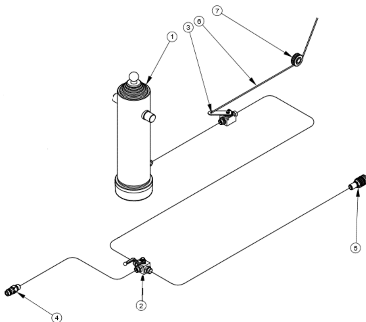
Rysunek 10. Schemat instalacji hydraulicznej mechanizmu przechylenia skrzyni ładunkowej:
