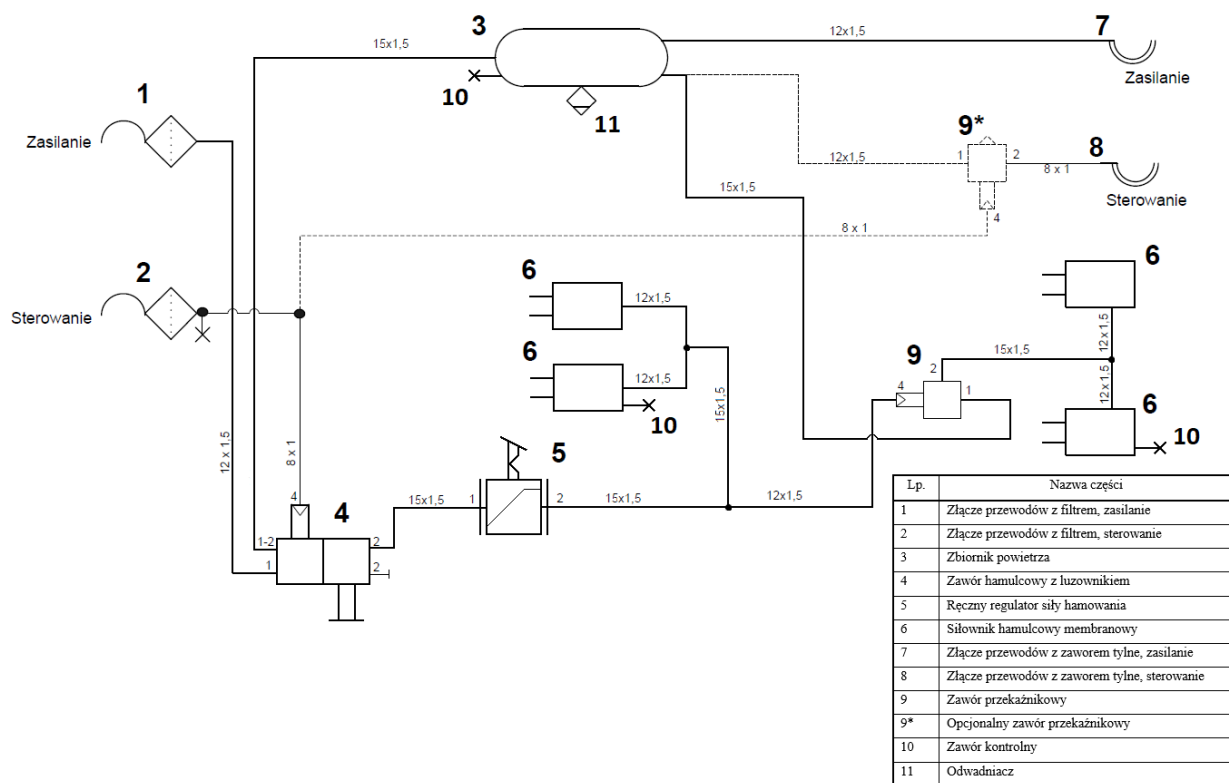
Rysunek 19. Schemat instalacji pneumatycznej dwuprzewodowej – regulator ręczny z zaworem przekaźnikowym (dwa siłowniki na oś)
