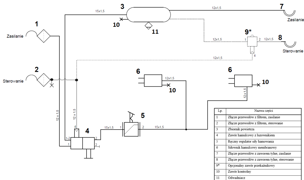
Rysunek 23. Schemat instalacji pneumatycznej dwuprzewodowej – regulator ręczny z zaworem przełącznikowym (jeden siłownik na oś)
