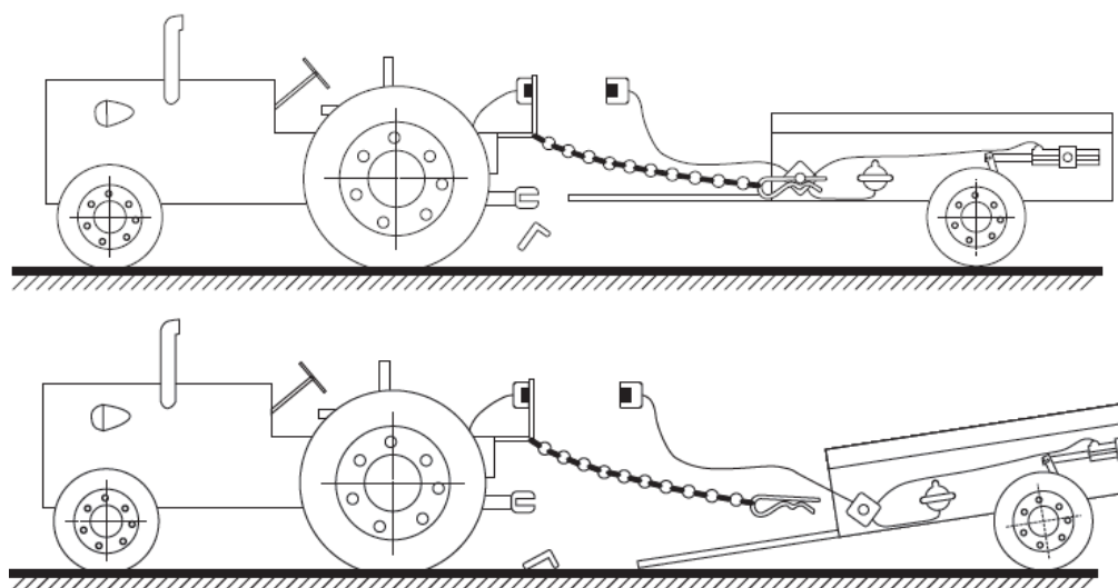
Rysunek 28. Schemat ilustrujący hamowanie awaryjne
