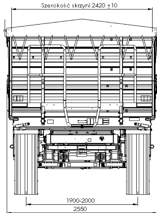
Rysunek 11. Wymiary przyczepy T711/L – widok z przodu
