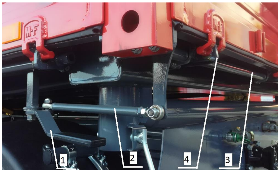
Rysunek 32. Zamki ścian skrzyni ładunkowej: 1- dźwignia centralna zamków dolnych, 2- mechanizm regulacji zamków, 3- centralny wałek zamków, 4-zamek
