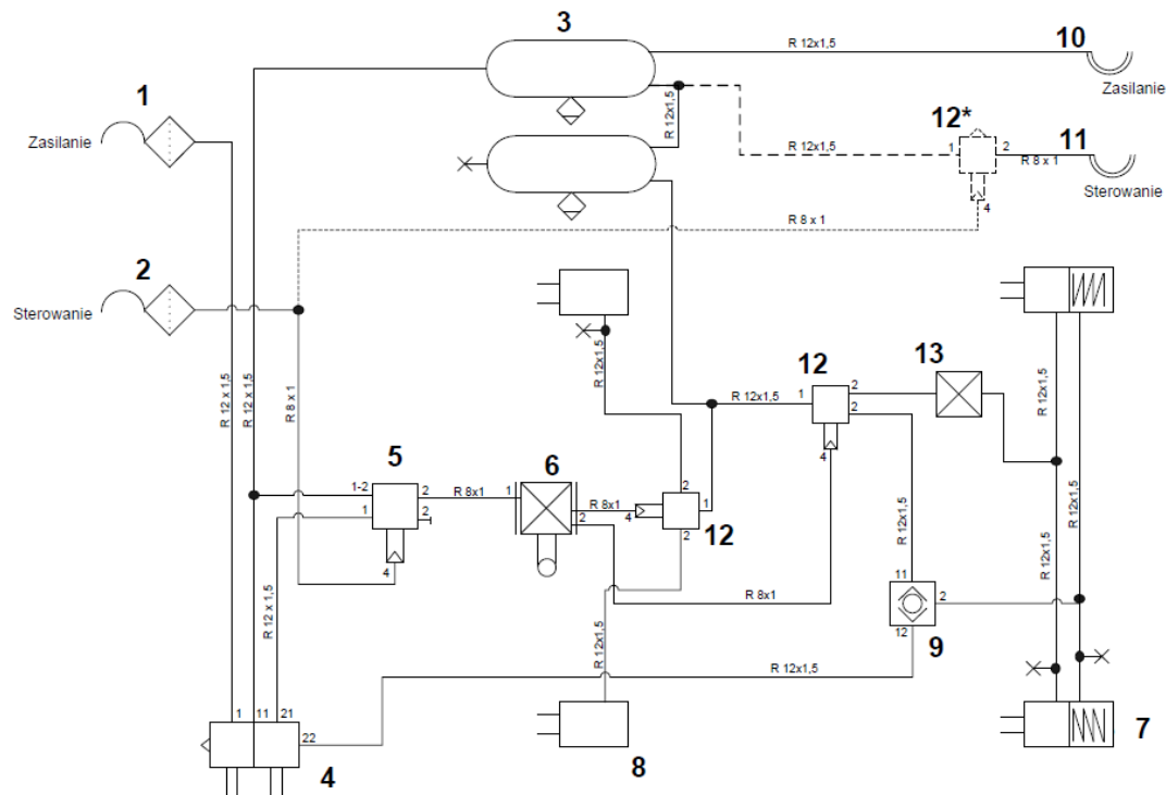
Rysunek 20. Schemat instalacji pneumatycznej dwuprzewodowej – ALB z zaworem przełącznikowym (dwa siłowniki na oś)
