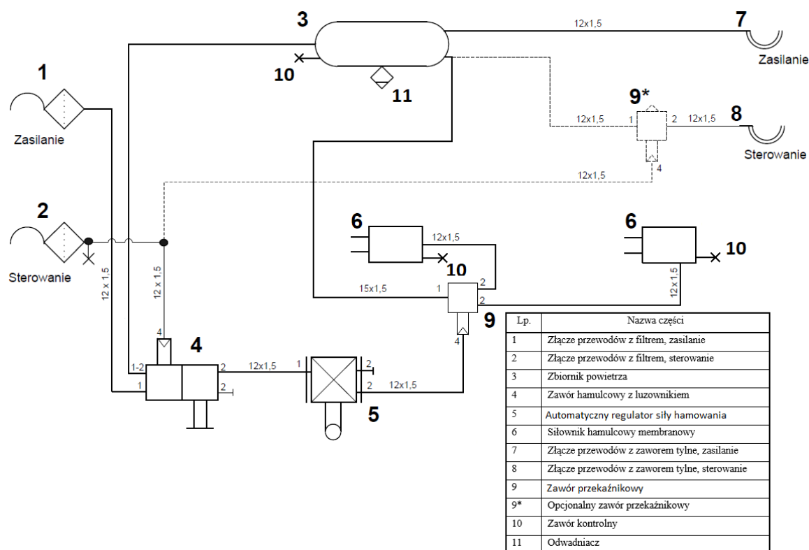
Rysunek 22. Schemat instalacji pneumatycznej dwuprzewodowej – ALB z zaworem przełącznikowym (jeden siłownik na oś)
