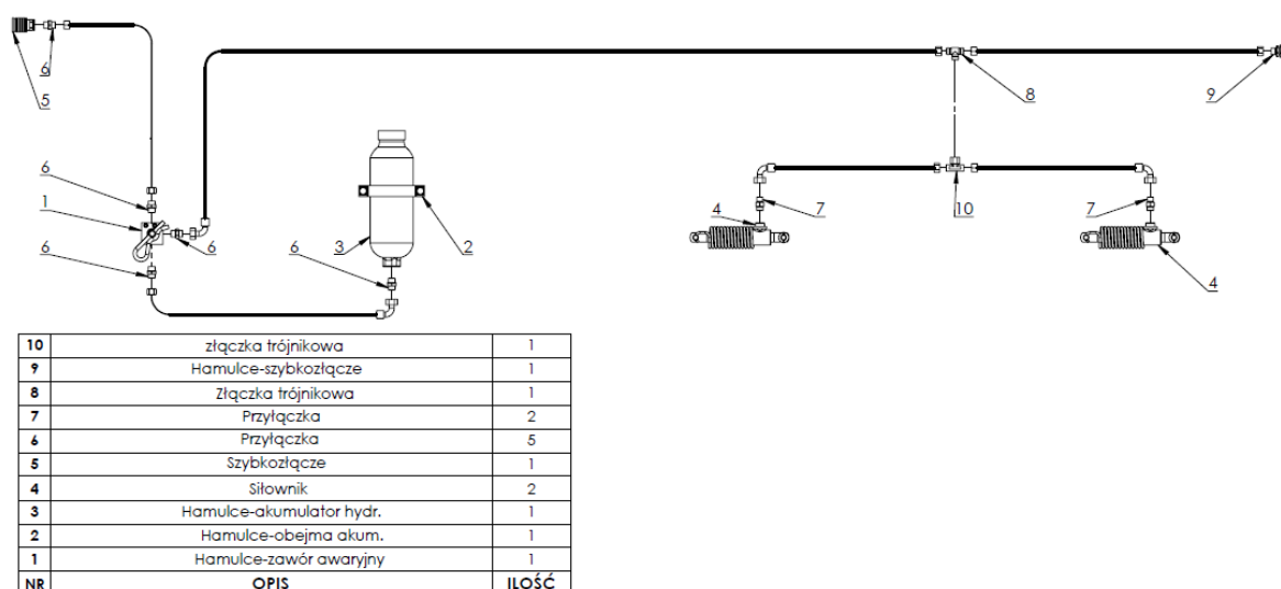
Rysunek 25. Schemat instalacji hydraulicznej jednoprzewodowej
