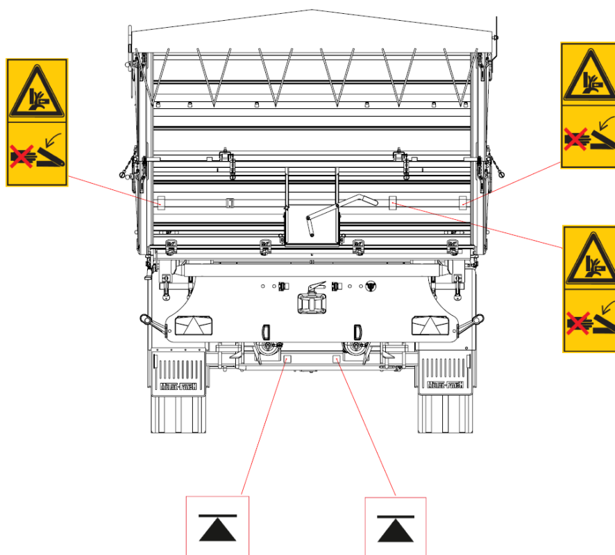
Rysunek 7. Rozmieszczenie piktogramów na ścianach przyczepy- tył
