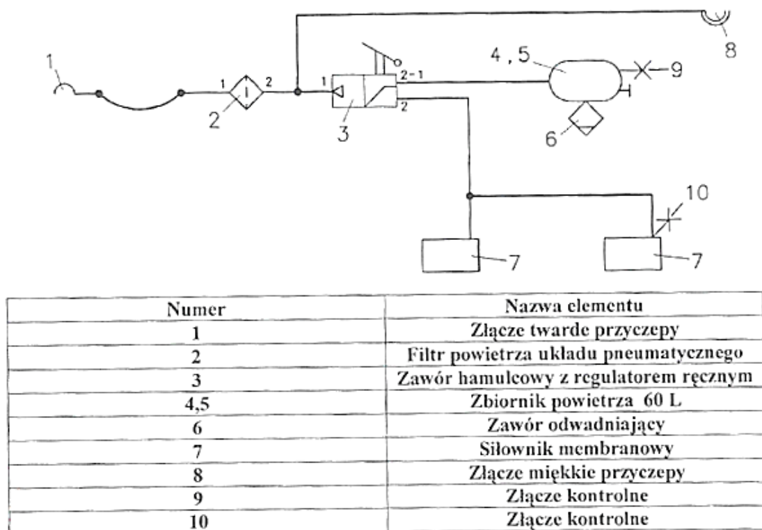
Rysunek 18. Schemat instalacji pneumatycznej jednoprzewodowej
