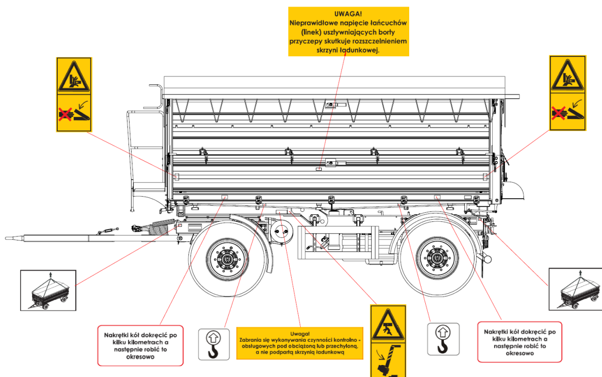
Rysunek 8. Rozmieszczenie piktogramów na ścianach przyczepy - lewa strona
