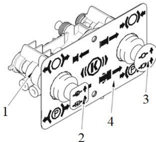
Rysunek 31. Hamulec postojowy – zawór luzująco parkujący. 1 – zawór, 2 – przycisk czerwony, 3 – przycisk czarny, 4 – tabliczka informacyjna
