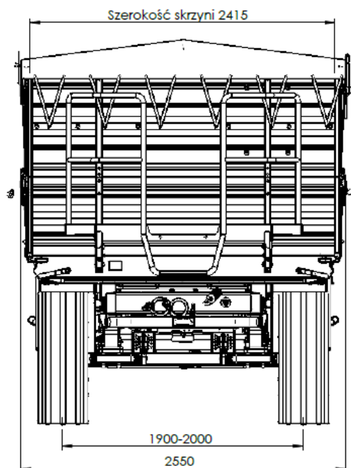
Rysunek 9. Wymiary przyczepy T711 – widok z przodu
