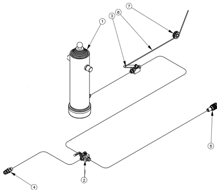
Rysunek 14. Schemat instalacji hydraulicznej mechanizmu przechylania skrzyni ładunkowej: 1 - siłownik teleskopowy, 2 – zawór przełączający, 3 - zawór odcinający, 4 –szybkozłącze - wtyczka, 5 – szybkozłącze – gniazdo, 6 - linka sterująca zaworem odcinającym, 7 –rolka linki
