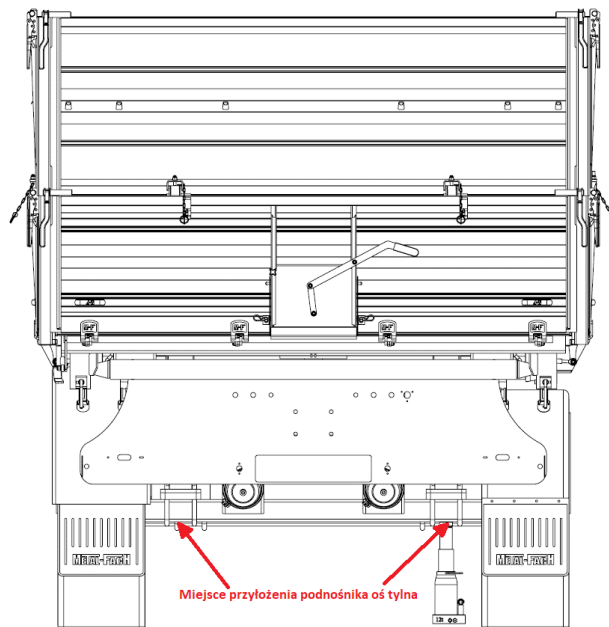
Rysunek 35. Punkty przyłożenia podnośnika – oś tylna
