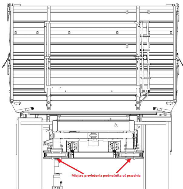
Rysunek 34. Punkty przyłożenia podnośnika – oś przednia
