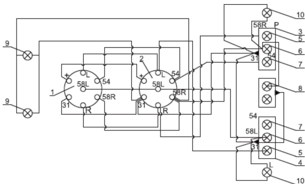
Rysunek 16. Schemat instalacji oświetleniowej bez światła pozycyjnych bocznych:
