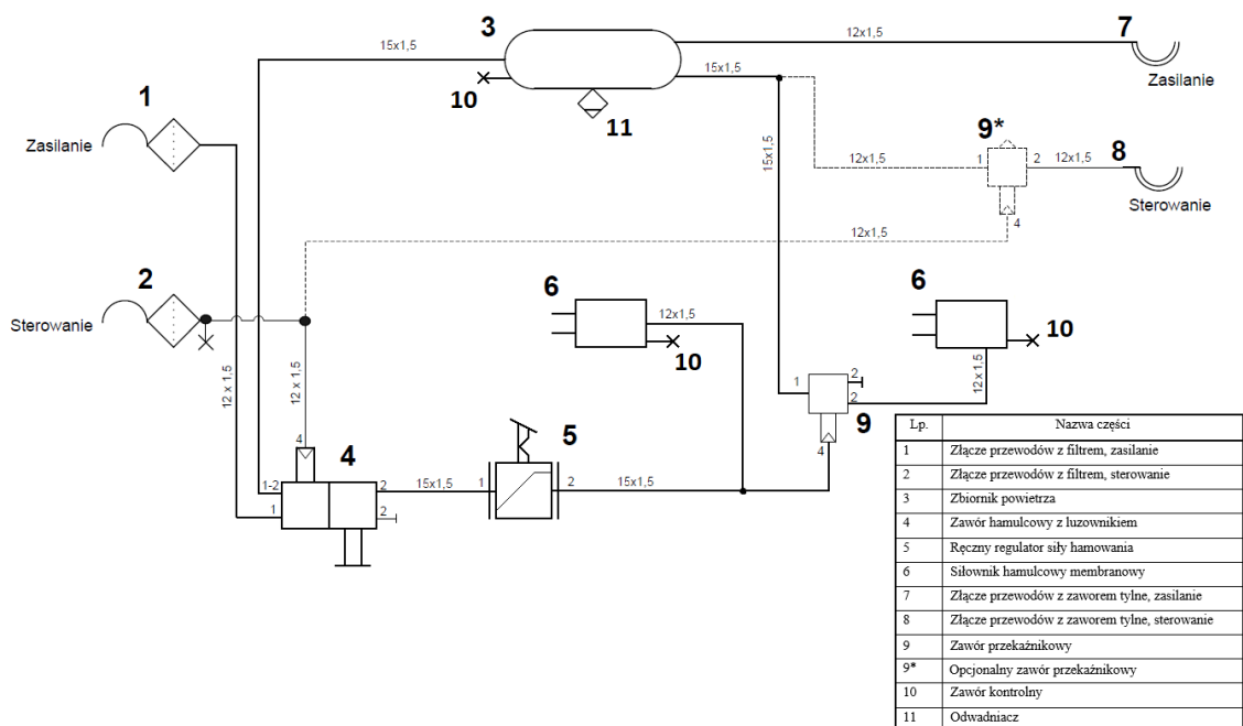
Rysunek 24. Schemat instalacji pneumatycznej dwuprzewodowej – regulator ręczny bez zaworu przełącznikowego ( jeden siłownik na oś)
