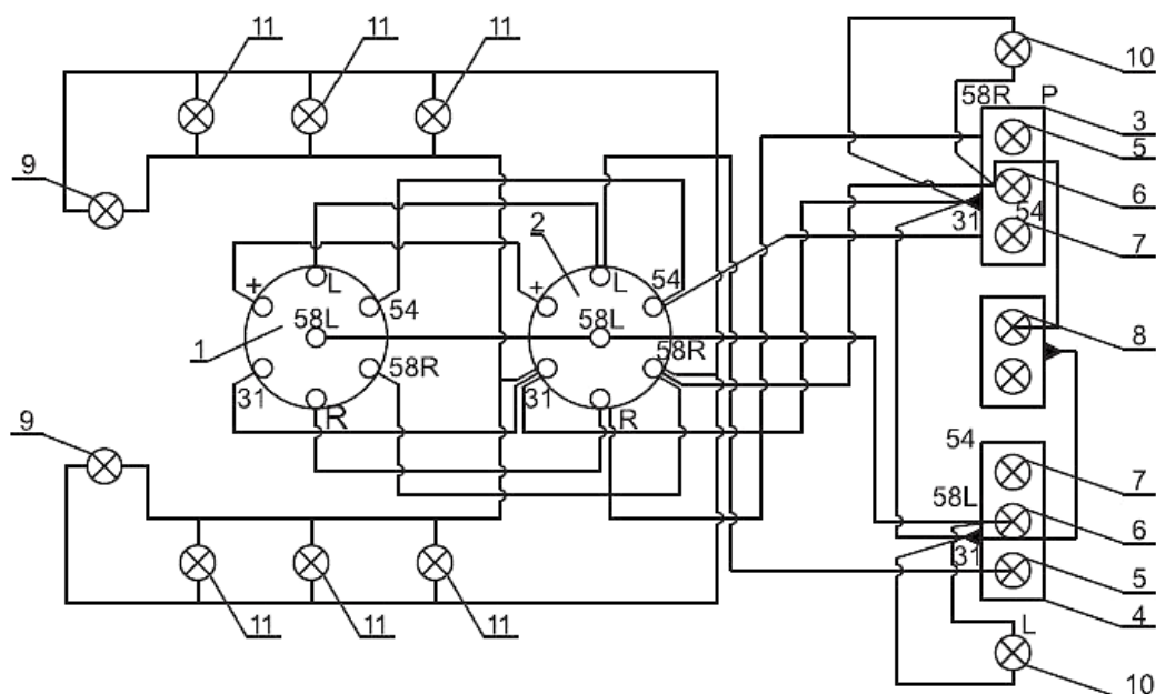
Rysunek 15. Schemat instalacji oświetleniowej zawierające światła pozycyjne boczne:
