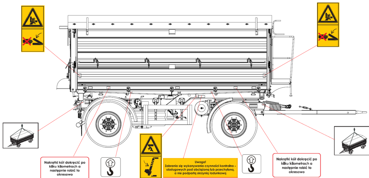
Rysunek 6. Rozmieszczenie piktogramów na ścianach przyczepy- prawa strona
