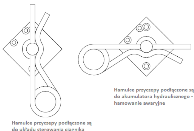
Rysunek 29. Ustawienie dźwigni zaworu bezpieczeństwa
