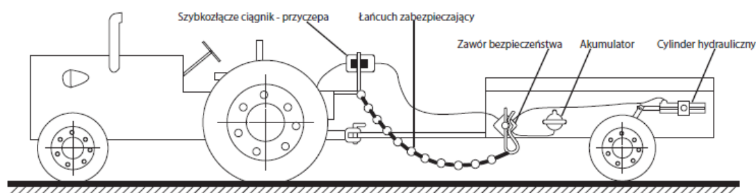
Rysunek 27. Prawidłowe połączenie ciągnik – przyczepa
