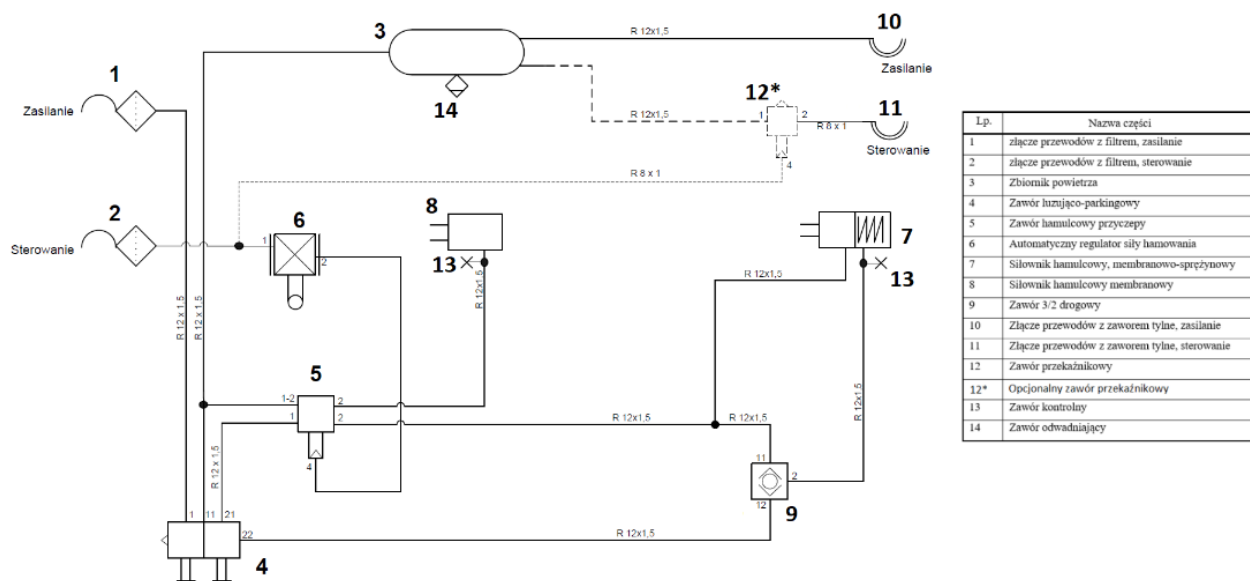
Rysunek 16. Układ hamulcowy z siłownikami membranowo - sprężynowymi bez zaworu przełącznikowego
