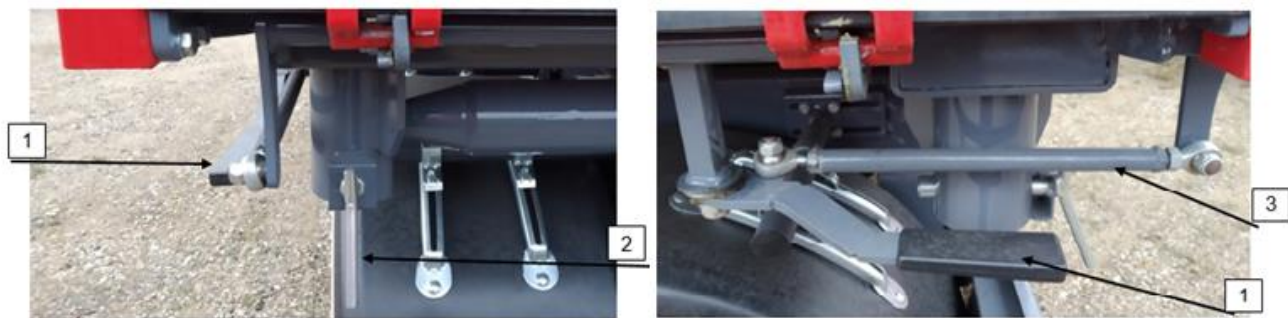
Rysunek 22. Zamki ścian skrzyni ładunkowej: 1- dźwignia centralna zamków dolnych, 2- zawleczka ustalająco -zabezpieczająca dźwigni, 3- dźwignia zamknięcia burt
