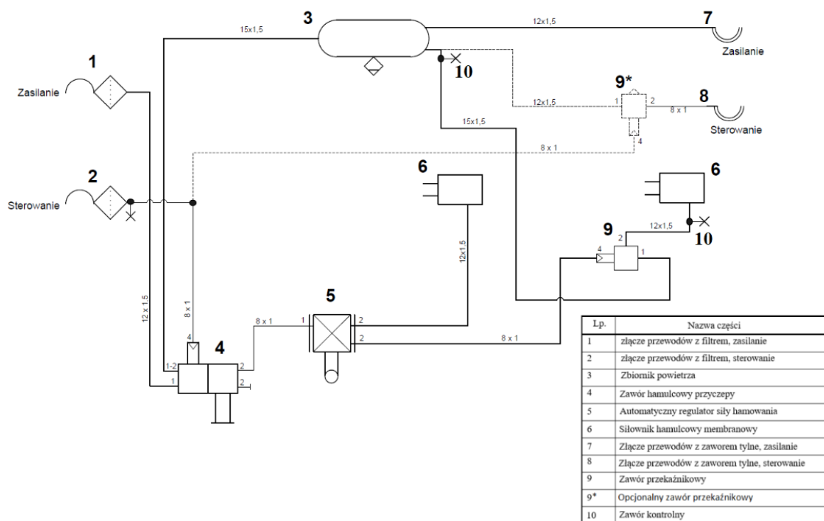
Rysunek 18. Układ hamulcowy ALB z zaworem przełącznikowym
