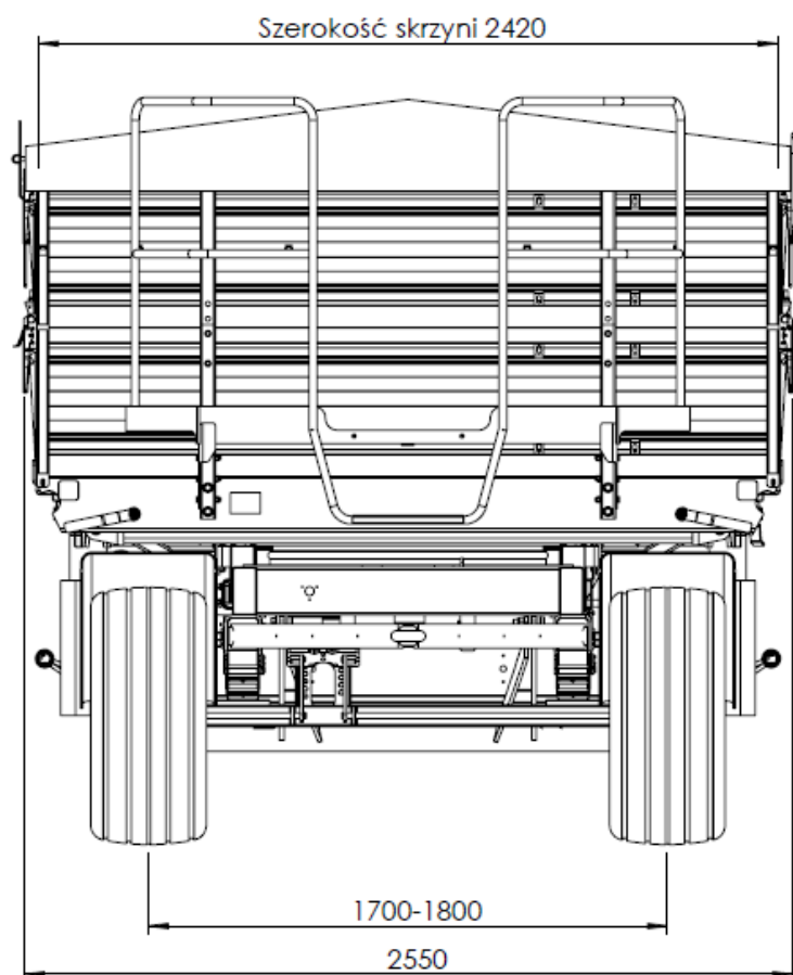
Rysunek 9. Wymiary przyczepy – widok z przodu
