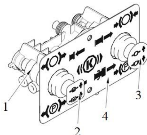
Rysunek 21. Hamulec postojowy – zawór luzująco parkujący:
