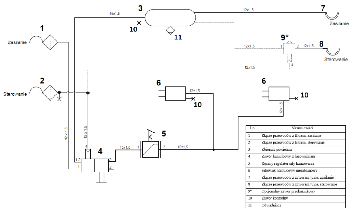
Rysunek 19. Układ hamulcowy z ręcznym regulatorem bez zaworu przełącznikowego
