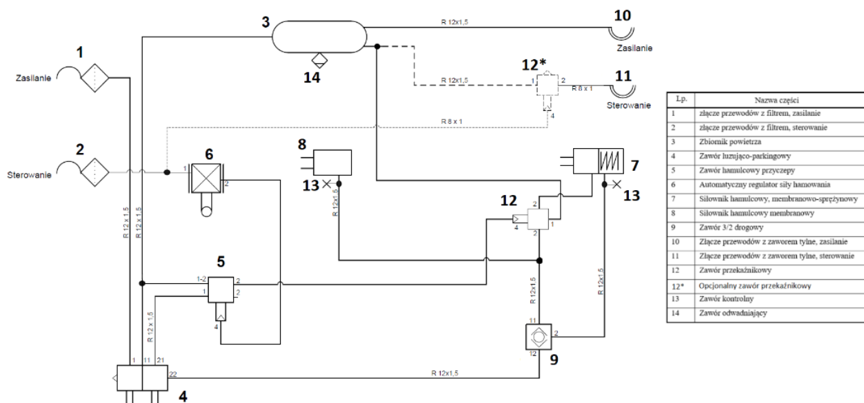
Rysunek 15. Układ hamulcowy z siłownikami membranowo - sprężynowymi i zaworem przełącznikowym
