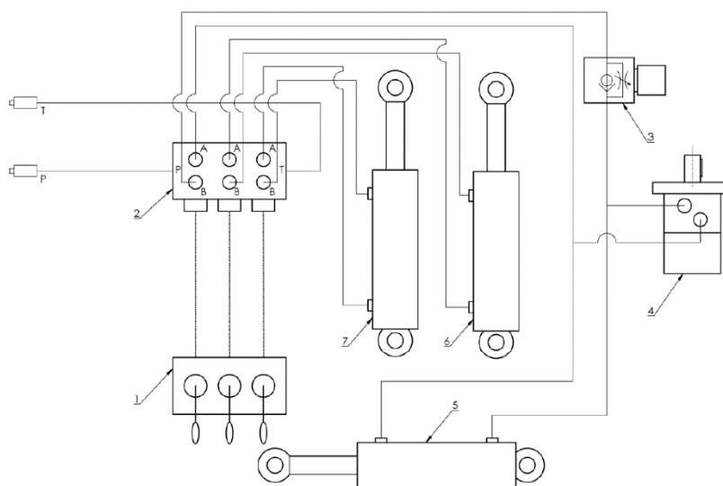
Rysunek 14. Układ hydrauliczny owijarki Z237 z mechanicznym obcinaczem folii
