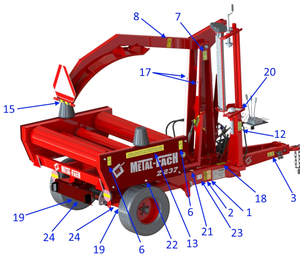
Rysunek 8. Rozmieszczenie piktogramów – strona prawa
