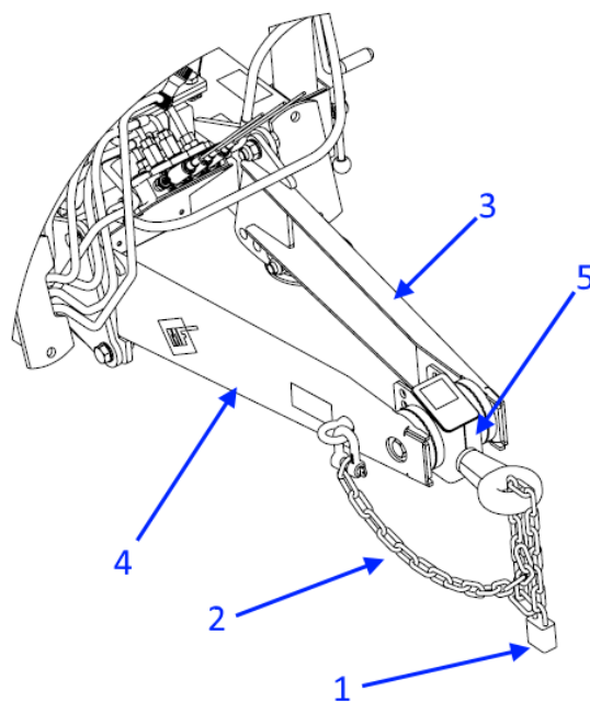
Rysunek 11. Wyposażenie dyszla
