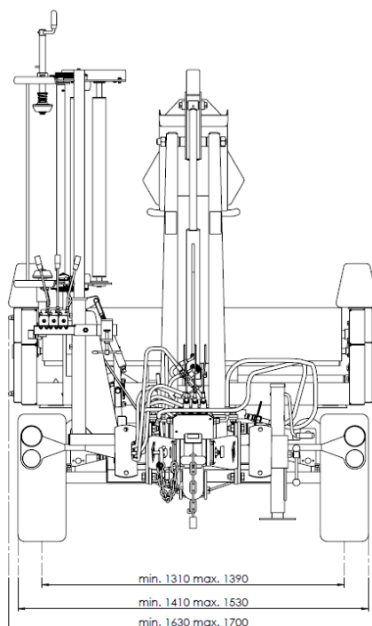
Rysunek 5. Wymiary owijarki – przód
