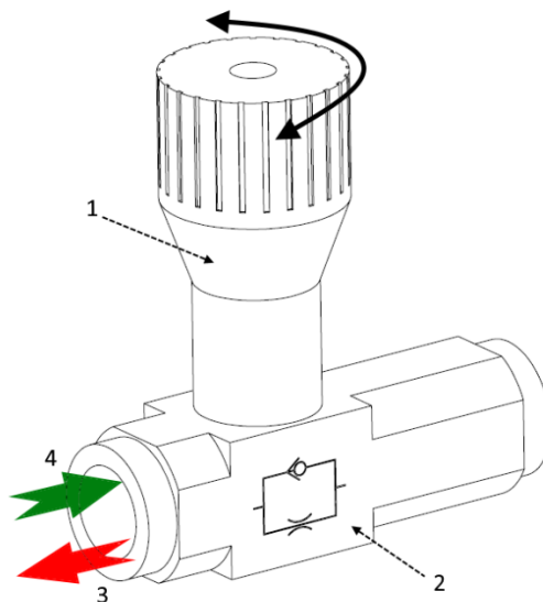
Rysunek 28. Zawór zwrotno-dławiący, 1 – pokrętło zaworu, 2 – korpus zaworu z oznaczeniem kierunku dławienia, 3 – kierunek przepływu dławiony, 4 – kierunek przepływu swobodny
