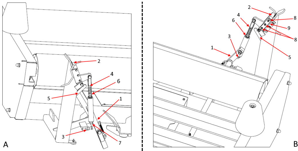
Rysunek 30. Obcinacz zamknięty: A – widok z przodu, B – widok z tyłu
