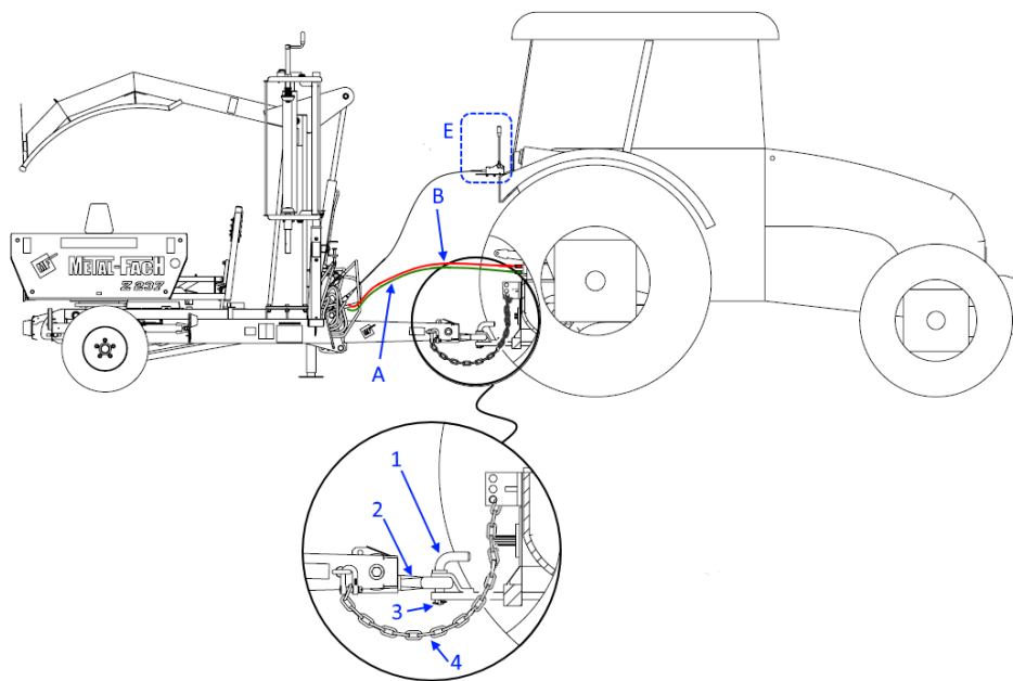
Rysunek 9. Schemat podłączenia zaczepu i napędu owijarki
