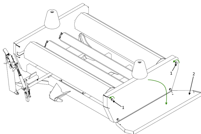
Rysunek 23. Demontaż osłony przekładni napędu bębnow
