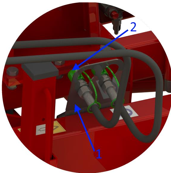
Rysunek 10. Miejsce przechowywania przewodów hydraulicznych: 1 – uchwyt przewodów, 2 – plastikowa nakładka
