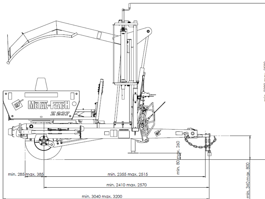
Rysunek 6. Wymiary owijarki – bok
