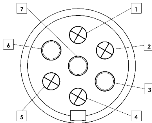
Rysunek 13. Wtyczka oświetleniowa owijkarki (widok od strony gniazda)
