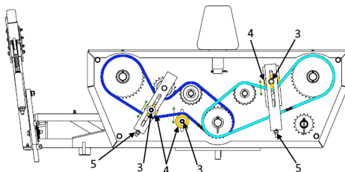
Rysunek 24. Regulacja napięcia łańcuchów napędu bębnow
