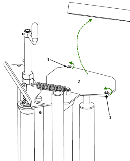
Rysunek 25. Demontaż osłony przekładni podajnika
