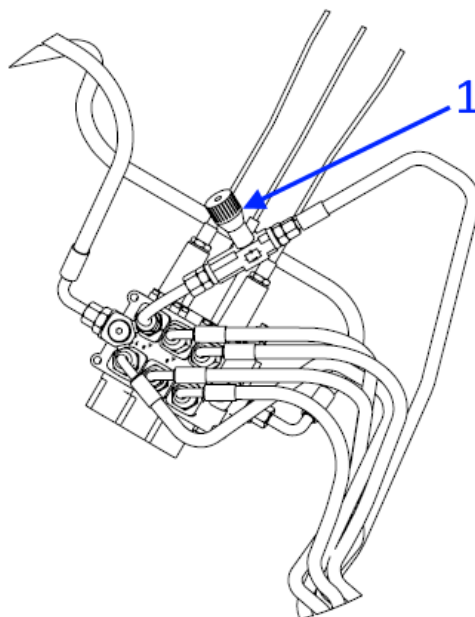
Rysunek 29. Umieszczenie zaworu regulacji blokady obrotu stołu roboczego
