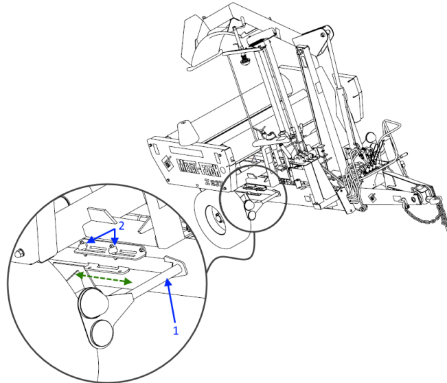
Rysunek 32. Pozycja transportowa oświetlenia przedniego
