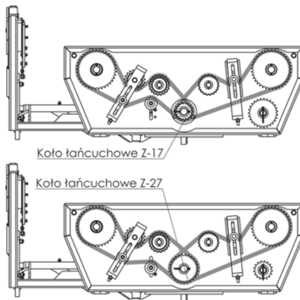
Rysunek 27. Koła łańcuchowe napędu bębnow
