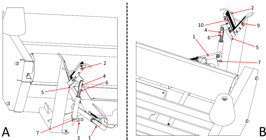
Rysunek 31. Obcinacz otwarty: A – widok z tyłu, B – widok z przodu
