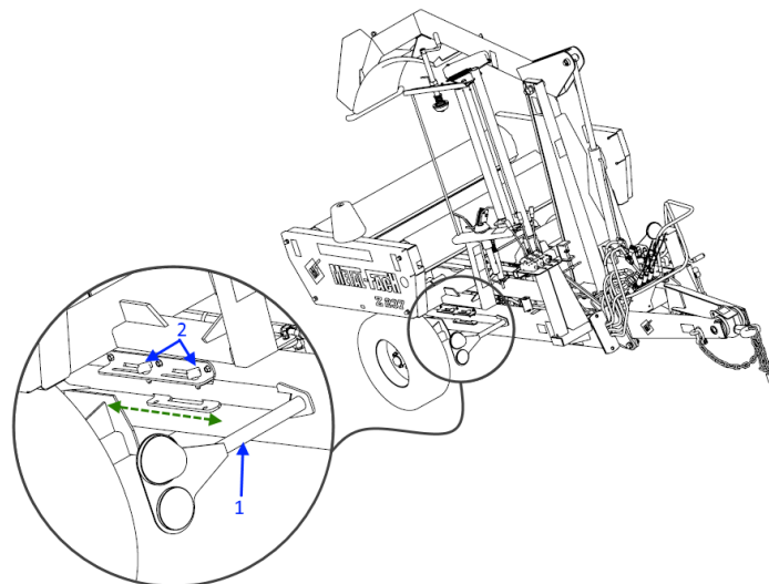
Rysunek 33. Pozycja robocza oświetlenia przedniego
