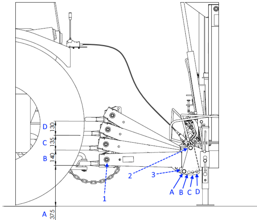
Rysunek 20. Regulacja wysokości zaczepu
