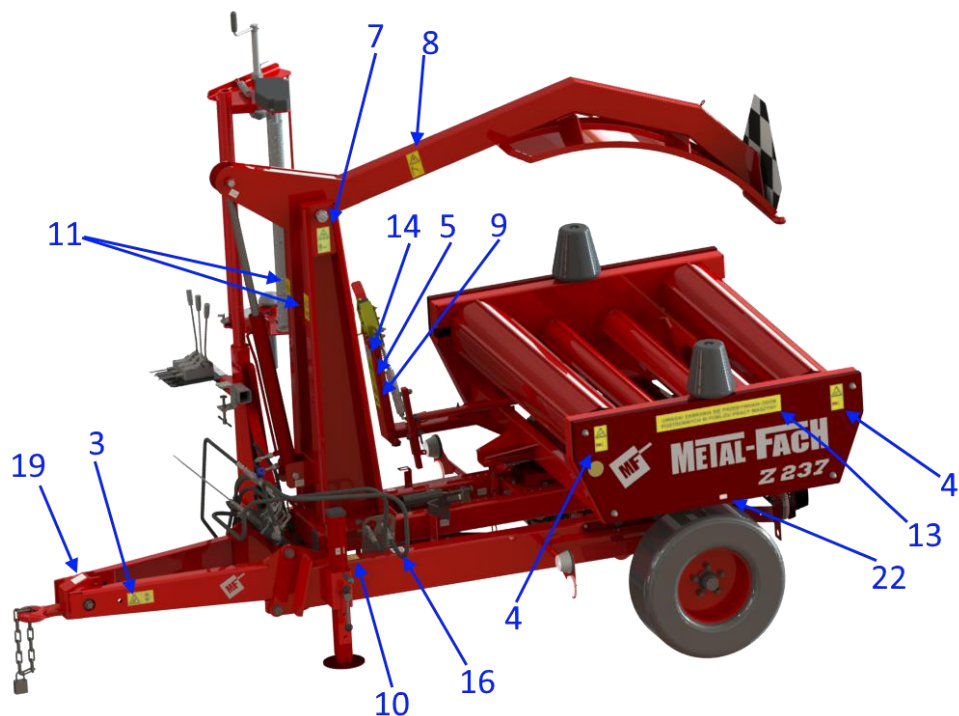
Rysunek 7. Rozmieszczenie piktogramów – strona lewa
