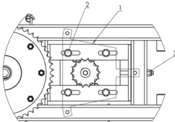
Rysunek 22. Regulacja łańcucha napędowego 1 – osłona łańcucha, 2 – nakrętki M12, 3 – śruba napinacza łańcucha.
