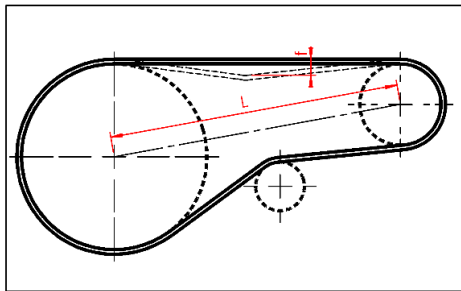
Rysunek 21. Regulacja napięcia łańcucha – wyznaczanie ugięcia łańcucha: f – wartość ugięcia łańcucha, L – odległość od środków osi kół łańcuchowych
