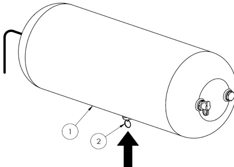
Rysunek 40. Odwadnianie zbiornika powietrza: 1 - zbiornik powietrza, 2 - zawór odwadniający
