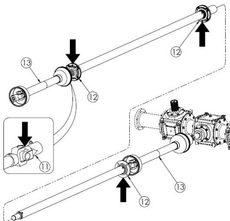
Rysunek 34. Punkty smarne rozrzutnika
