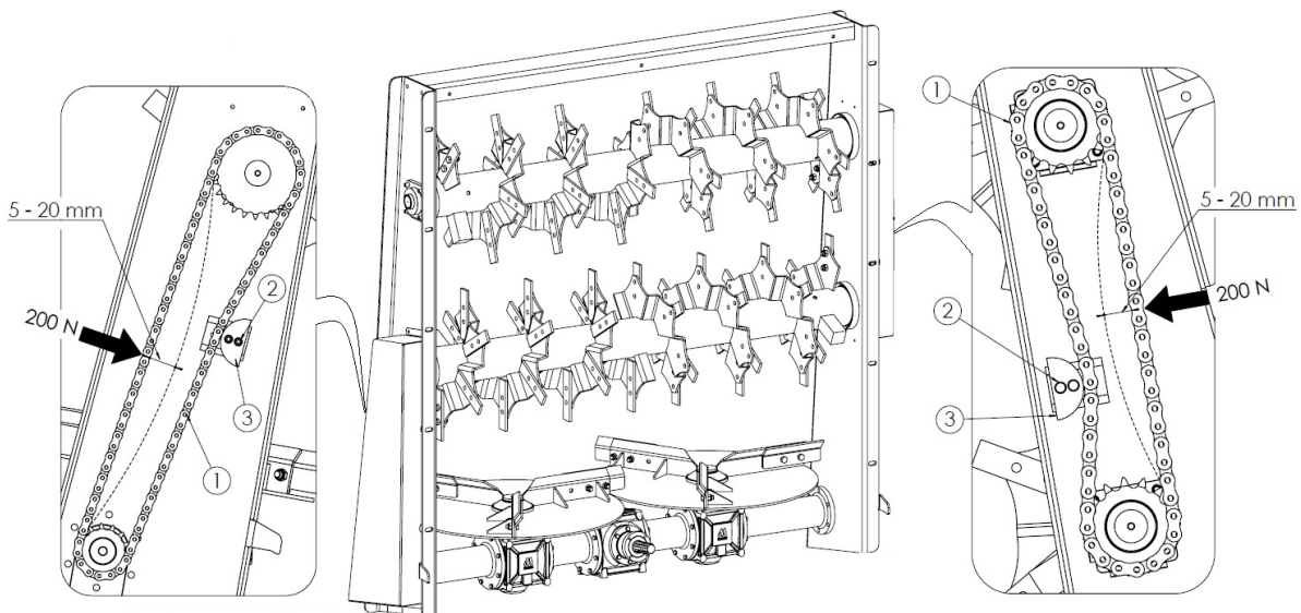
Rysunek 29. Napinanie łańcuchów adaptera
