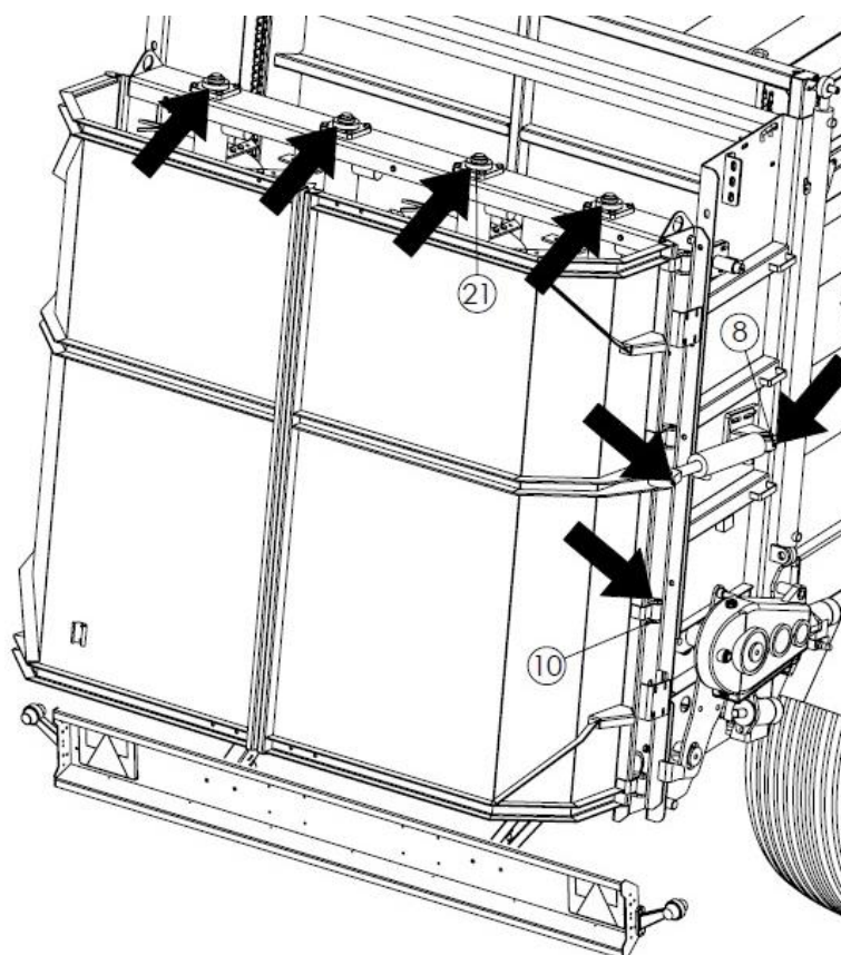
Rysunek 37. Punkty smarne rozrzutnika (adapter pionowy 4-wirnikowy)
