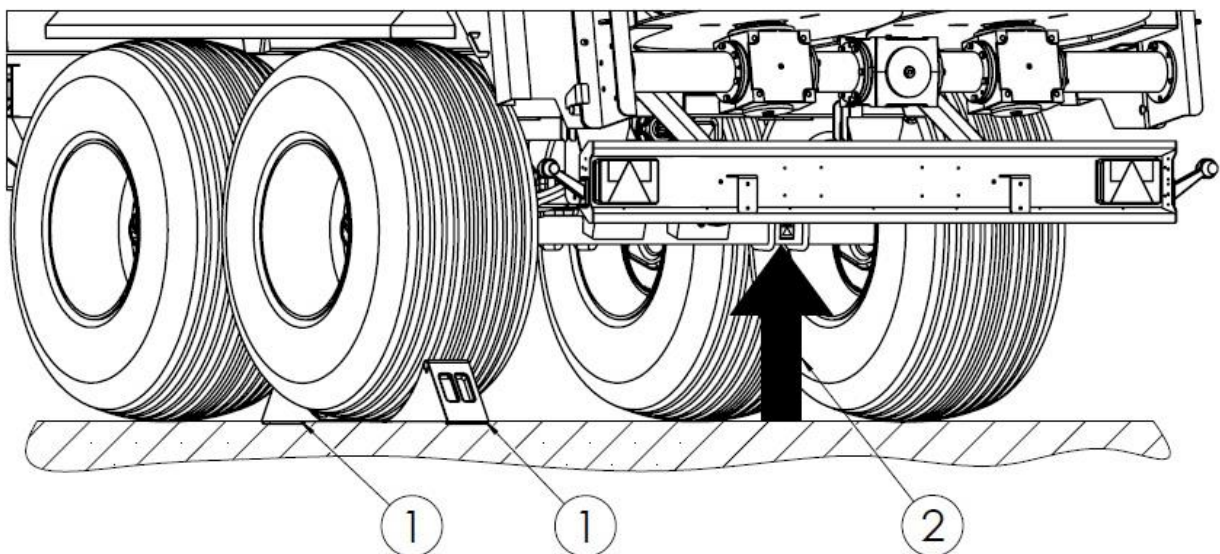
Rysunek 44. Punkty przyłożenia podnośników 1 - kliny, 2 - podnośnik
