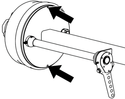
Rysunek 42. Kontrola zużycia okładzin hamulców
