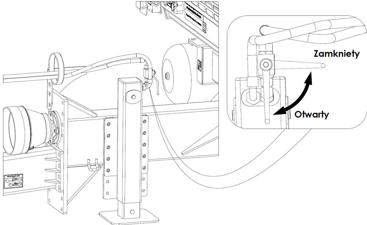
Rysunek 20. Zawór hydrauliczny sterujący (odcinający) stopkę hydrauliczną
