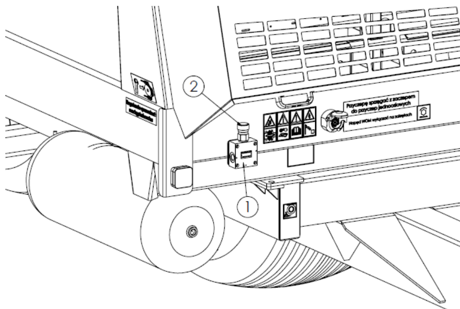
Rysunek 24. Regulacja prędkości przesuwu przenośnika podłogowego 1 - regulator przyływu oleju, 2 - pokrętko regulatora
