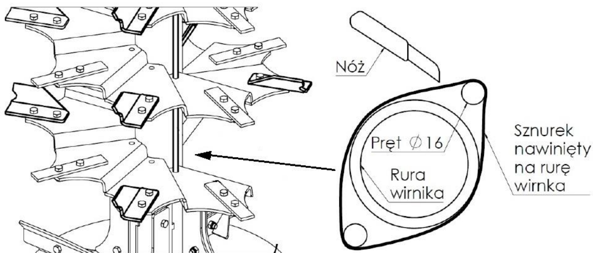
Rysunek 46. Czyszczenie nawiniętych sznurków, siatek
