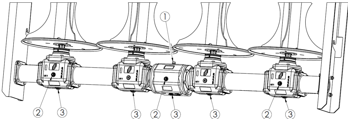
Rysunek 32. Punkty kontroli poziomu oleju przekładni adaptera pionowego 4-wirnikowego 1 - wlew oleju (odpowietrznik), 2 - wznik poziomu oleju, 3 - korki spustowe
