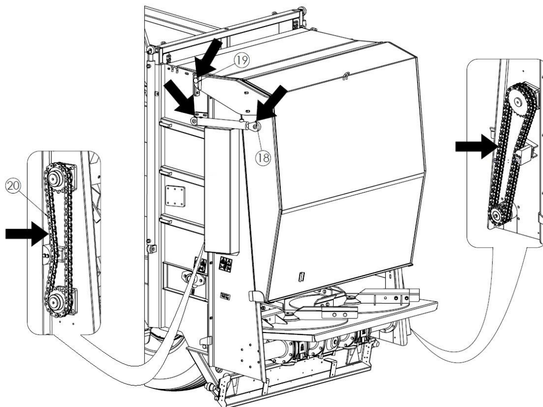
Rysunek 36. Punkty smarne rozrzutnika (adapter tarczowo-poziomy 2-wirnikowy)
