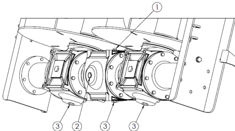
Rysunek 31. Punkty kontroli poziomu oleju przekładni adaptera pionowego 2-wirnikowego i adaptera trczowo-poziomego 2-wirnikowego 1 - wlew oleju (odpowietrznik), 2 - wznik poziomu oleju, 3 - korki spustowe
