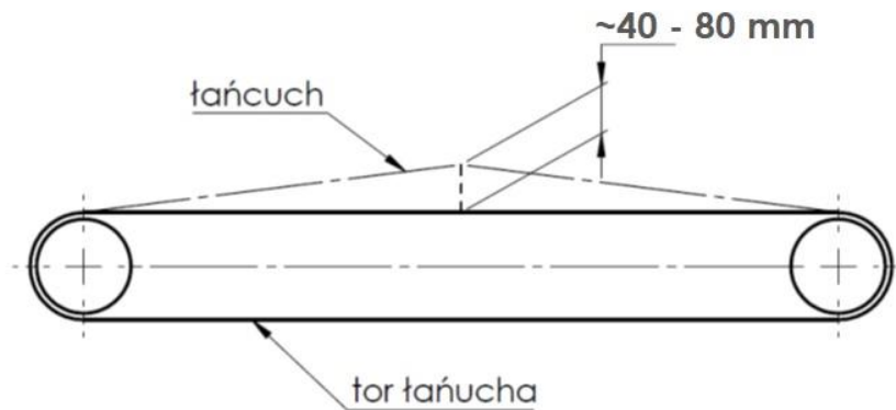
Rysunek 28. Sprawdzenie naciągu łańcucha w rozrzutniku
