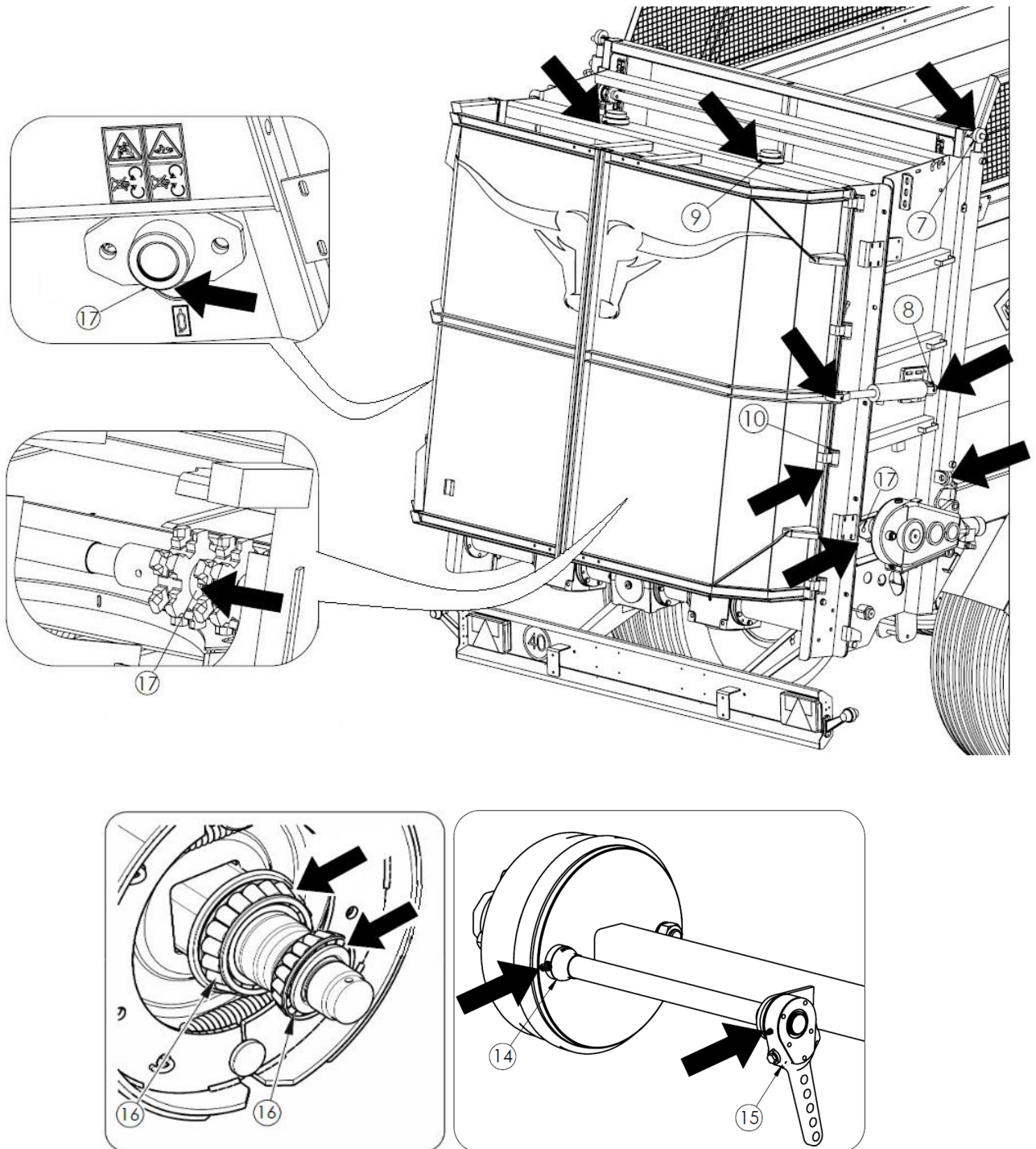
Rysunek 35. Punkty smarne rozrzutnika
