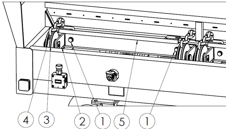
Rysunek 27. Napinanie łańcuchów przenośnika podłogowego 1 - śruba regulacyjna, 2 – suwak napinacza, 3- rolka napinacza, 4 – łańcuch przenośnika, 5 – listwa przenośnika
