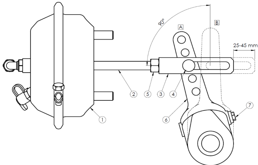
Rysunek 43. Regulacja hamulca zasadniczego
