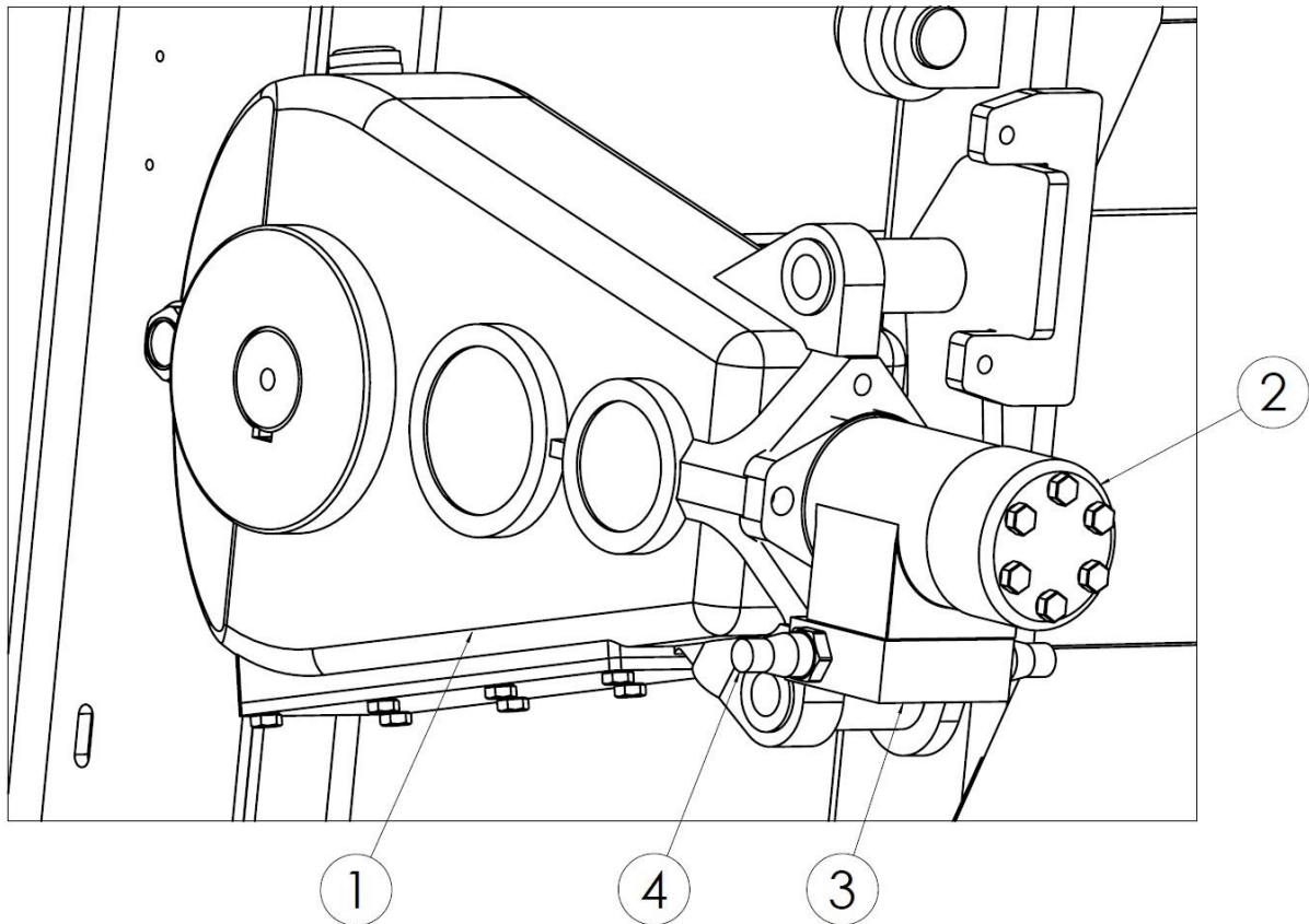
Rysunek 26. Napęd przenośnika podłogowego
