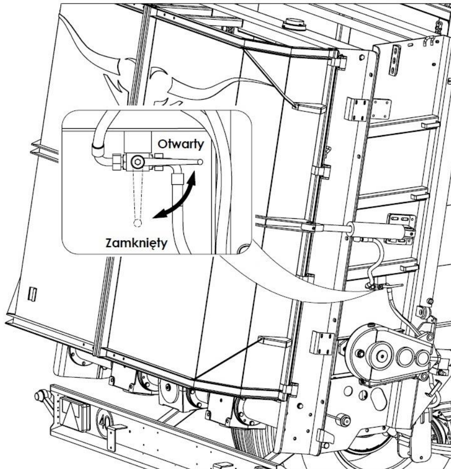
Rysunek 25. Zawór hydrauliczny blokujący osłonę adaptera
