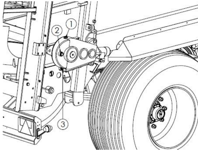
Rysunek 30. Punkty kontroli poziomu oleju przekładni przenośnika podłogowego 1 - wlew oleju (odpowietrznik), 2 - wznik poziomu oleju, 3 - korek spustowy
