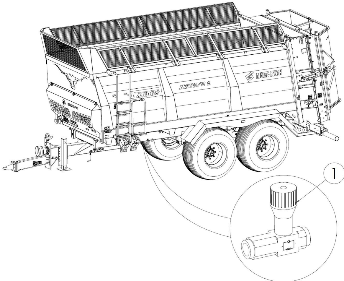
Rysunek 33. Regulator otwierania kłapy
