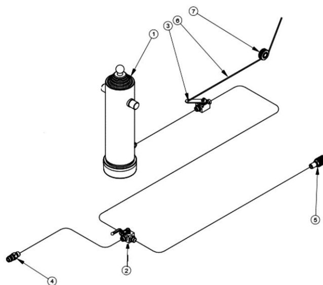
Rysunek 7. Schemat instalacji hydraulicznej mechanizmu przechylania skrzyni ładunkowej,
