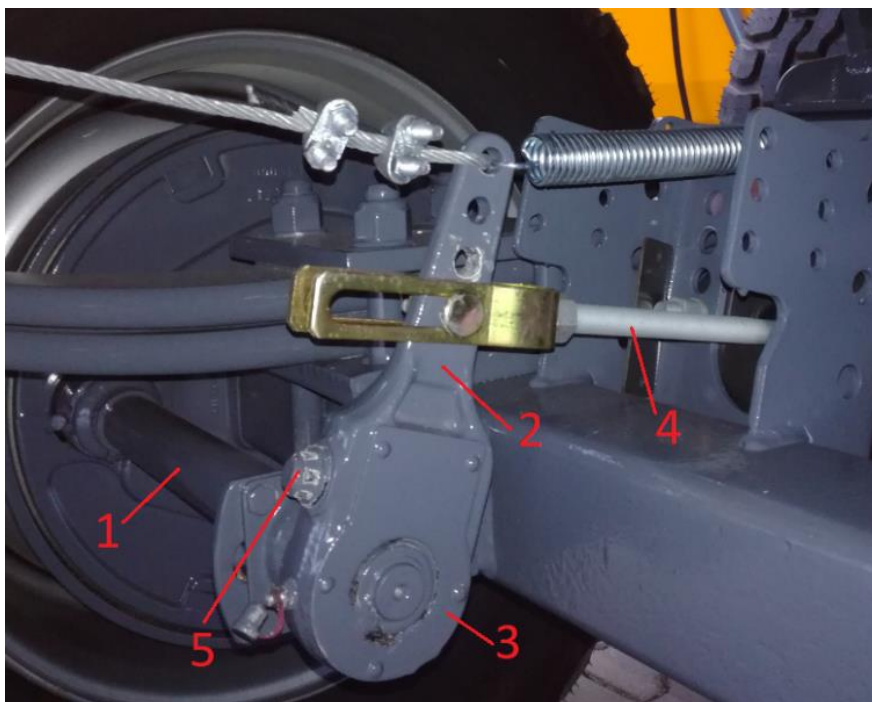
Rysunek 5. Elementy układu hamulcowego: 1-walek rozpieraka szczęk, 2-dźwignia (ramię) wałka rozpieraka, 3-zębatka na wałku rozpieraka, 4-ciężno (popychacz) łączące tłoczysko siłownika pneumatycznego z ramieniem wałka rozpieraka, 5 - śruba regulacji
