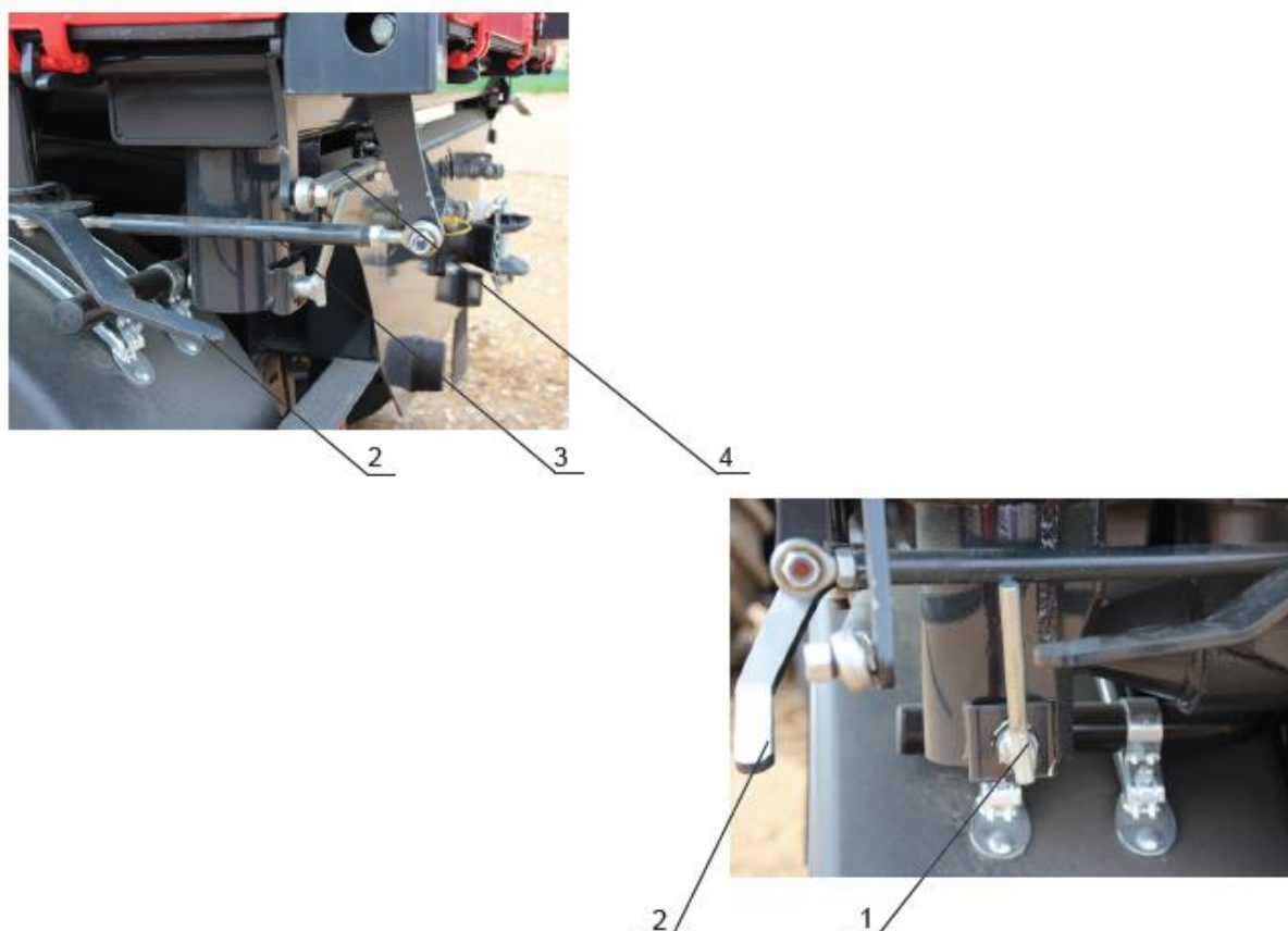
Rysunek 8. Zamki ścian skrzyni ładunkowej.
