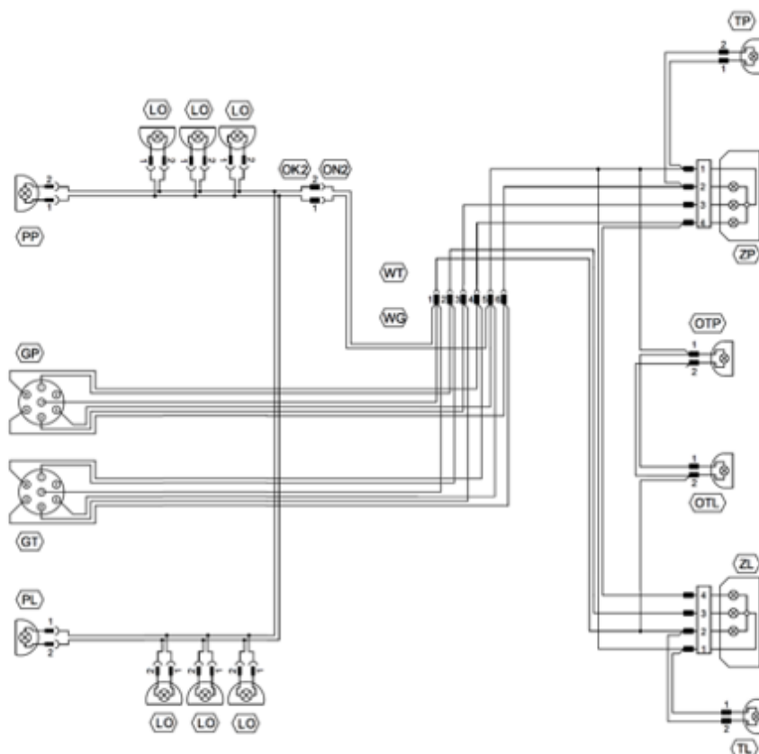
Rysunek 9. Schemat instalacji elektrycznej przyciepy:
