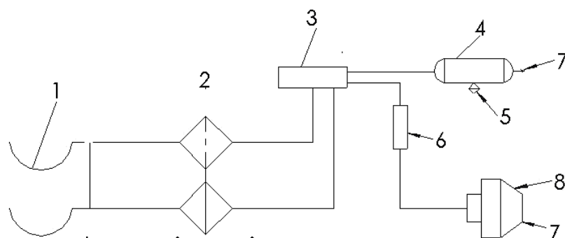
Рисунок 12. Схема однопроводной пневматической системы Т735А
