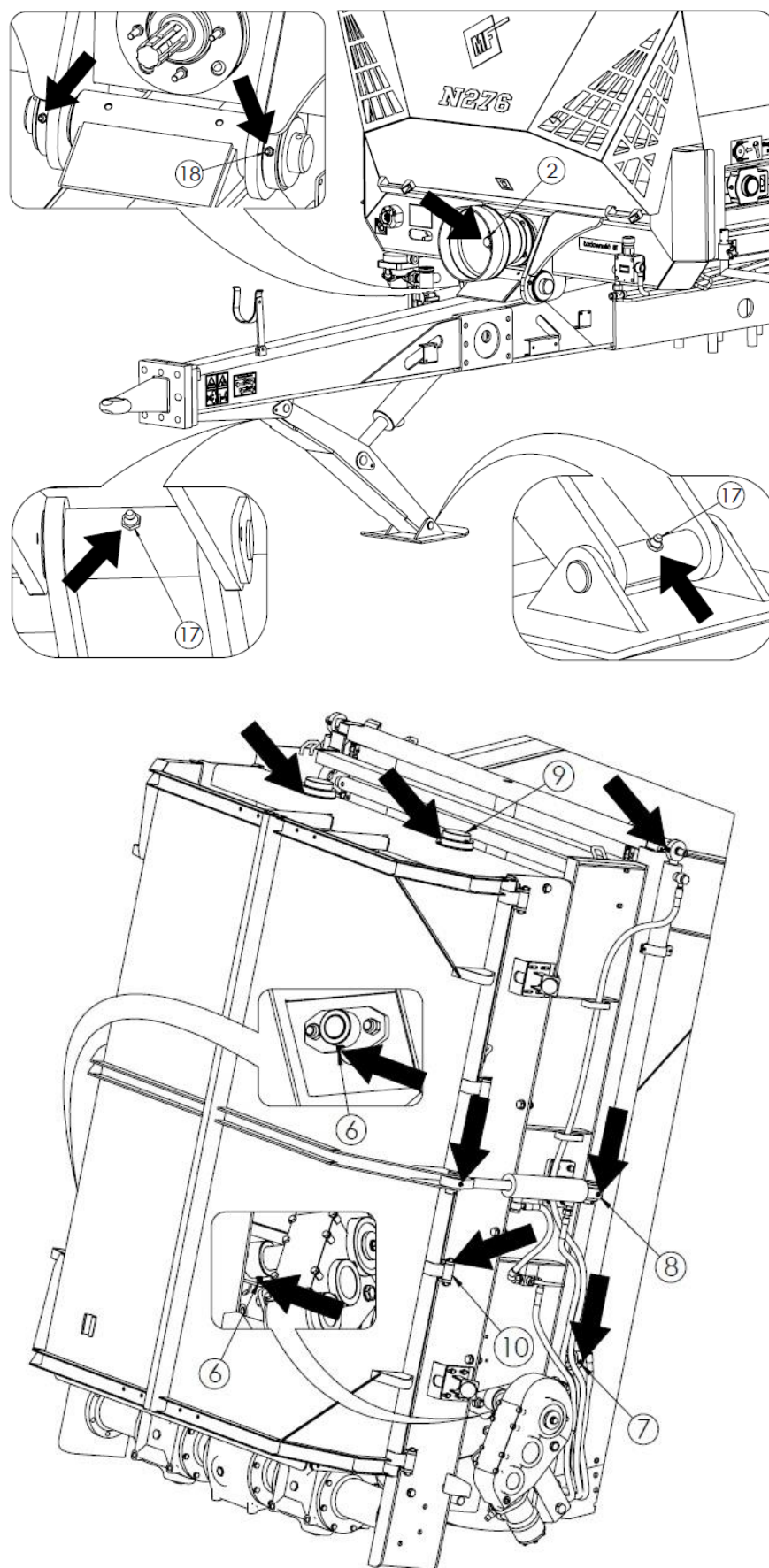
Rysunek 23. Punkty smarne
