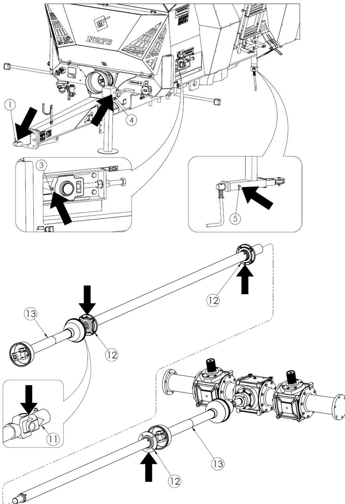
Rysunek 22. Punkty smarne
