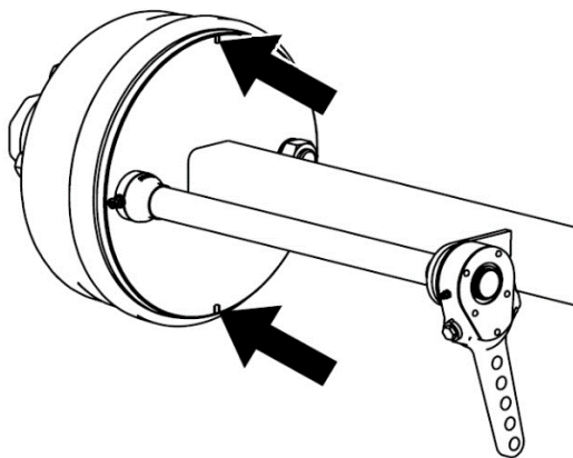
Rysunek 29. Kontrola zużycia okładzin hamulców
