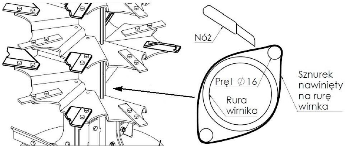
Rysunek 32. Czyszczenie nawiniętych sznurków, siatek
