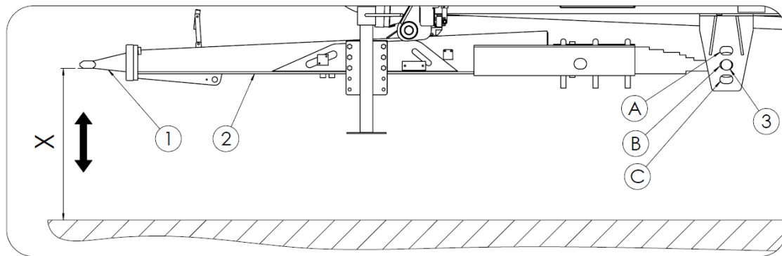
Rysunek 15. Położenie dyszla względem podłoża
