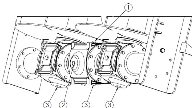
Rysunek 21. Punkty kontroli poziomu oleju przekładni adaptera. 1 - wlew oleju (odpowietrznik), 2 - wziernik poziomu oleju, 3 - korki spustowe
