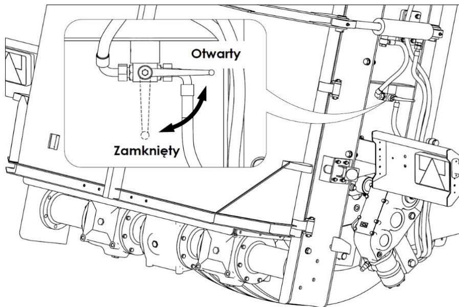
Rysunek 17. Zawór hydrauliczny blokujący osłonę adaptera (osłony otwierane hydraulicznie występują jako opcja wyposażenia)
