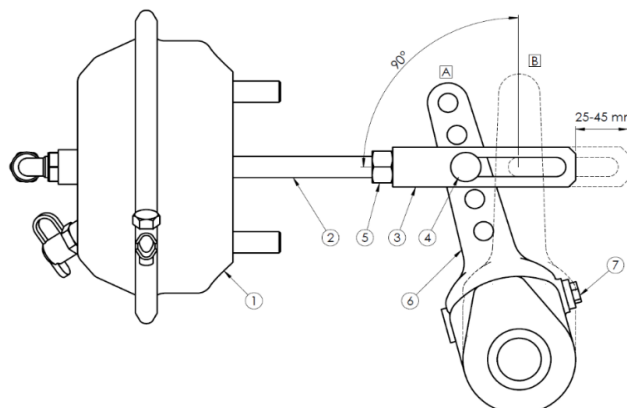
Rysunek 30. Regulacja hamulca zasadniczego
