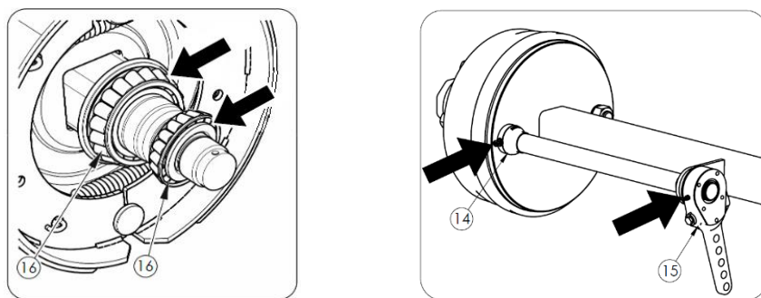
Rysunek 24. Punkty smarne
