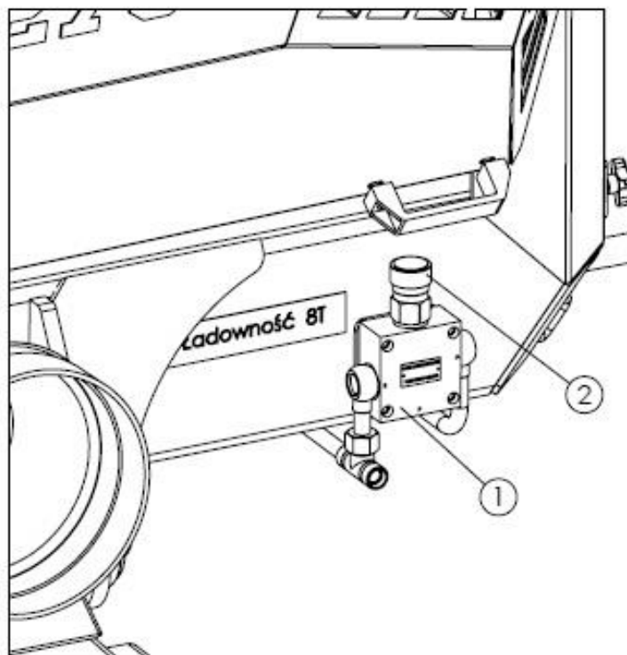
Rysunek 16. Regulacja prędkości przesuwu przenośnika podłogowego 1 - regulator przepływu oleju, 2 - pokrętło regulatora
