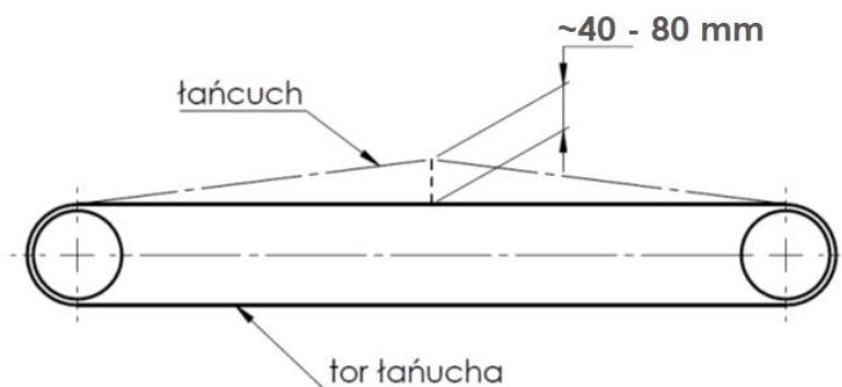
Rysunek 19. Sprawdzenie naciągu łańcucha w rozrzutniku
