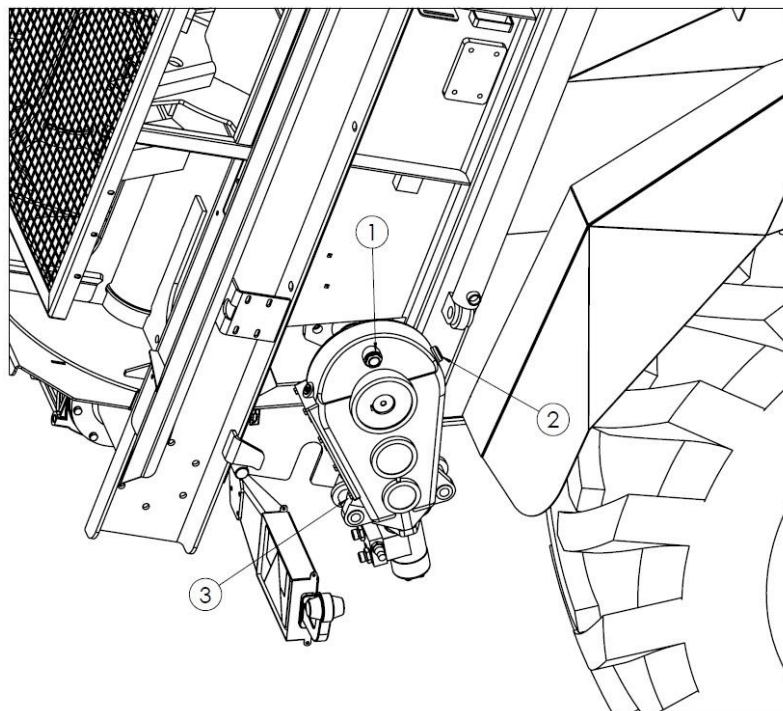
Rysunek 20. Punkty kontroli poziomu oleju przekładni przenośnika podłogowego. 1 - wlew oleju (odpowietrznik), 2 - wziernik poziomu oleju, 3 - korek spustowy
