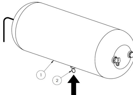
Rysunek 27. Odwadnianie zbiornika powietrza: 1 - zbiornik powietrza, 2 - zawór odwadniający
