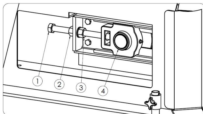
Rysunek 18. Napinanie łańcuchów przenośnika podłogowego 1 - śruba regulacyjna, 2-3 - nakrętki, 4 - zespół łożyskowy napinacza
